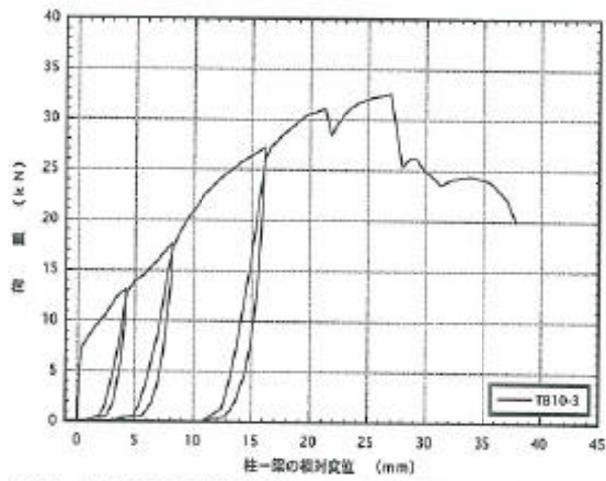
図4. 3 : TB10-3 梁受け金物DB-10の引張載荷試験の荷重-変位曲線
