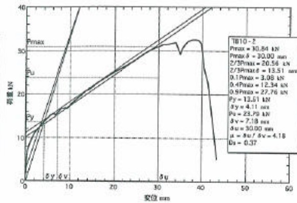
図5. 2 : TB10-2の荷重-変位包絡線
