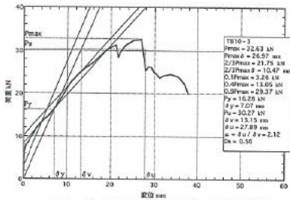
図5. 3 : TB10-3の荷重-変位包絡線
