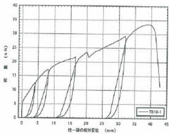
図4. 1 : TB10-1 梁受け金物DB-10の引張載荷試験の荷重-変位曲線
