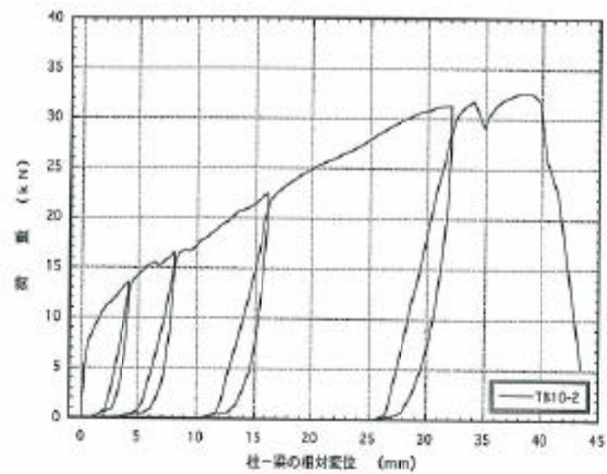
図4. 2 : TB10-2 梁受け金物DB-10の引張載荷試験の荷重-変位曲線
