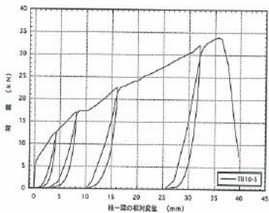
図4. 5 : TB10-5 梁受け金物DB-10の引張載荷試験の荷重-変位曲線
