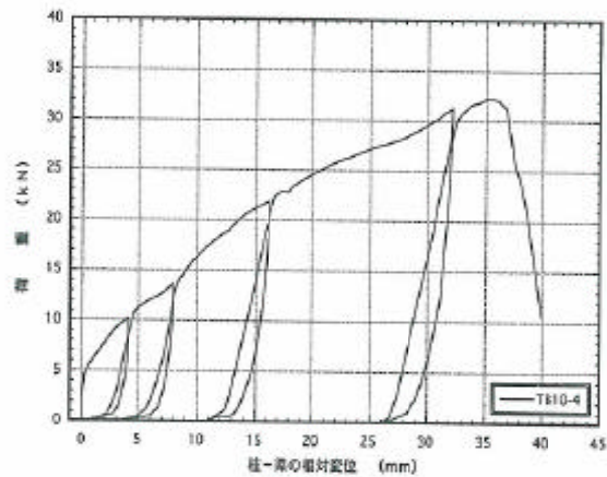
図4. 4 : TB10-4 梁受け金物DB-10の引張載荷試験の荷重-変位曲線
