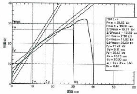
図5. 4 : TB10-4の荷重-変位包絡線
