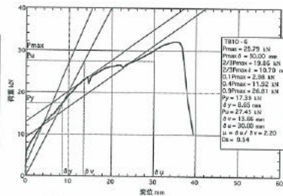
図5. 6 : TB10-6の荷重-変位包絡線
