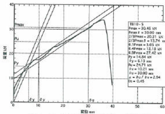
図5. 5 : TB10-5の荷重-変位包絡線
