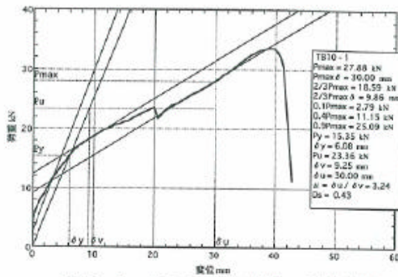
図5. 1 : TB10-1の荷重-変位包絡線
