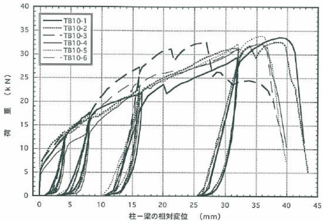
図4. 7 : TB10 梁受け金物DB-10の引張載荷試験の荷重-変位曲線
