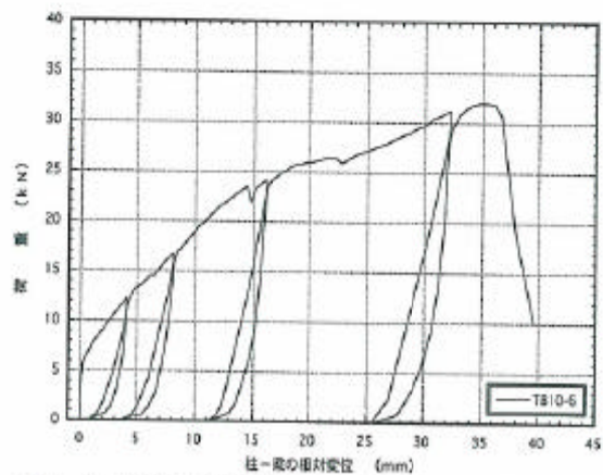
図4. 6 : TB10-6 梁受け金物DB-10の引張載荷試験の荷重-変位曲線
