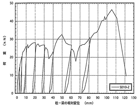
図4. 2 : SD10-2 梁受け金物DB-10のせん断荷試験の荷重-変位曲線
