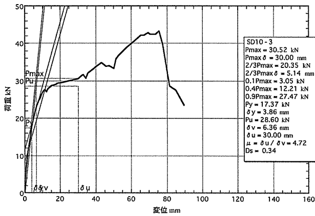
図5. 3 : SD10-3の荷重-変位包絡線
