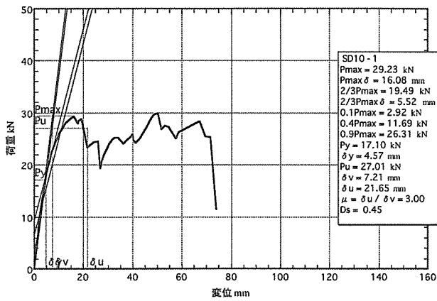
図5. 1 : SD10-1の荷重-変位包絡線
