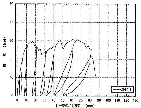
図4. 4 : SD10-4 梁受け金物DB-10のせん断荷試験の荷重-変位曲線
