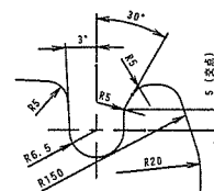
C部詳細図 (S=1/2)
