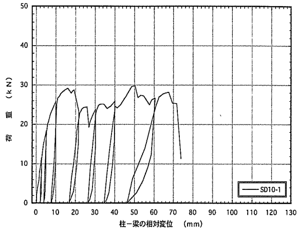
図4. 1 : SD10-1 梁受け金物DB-10のせん断荷試験の荷重-変位曲線
