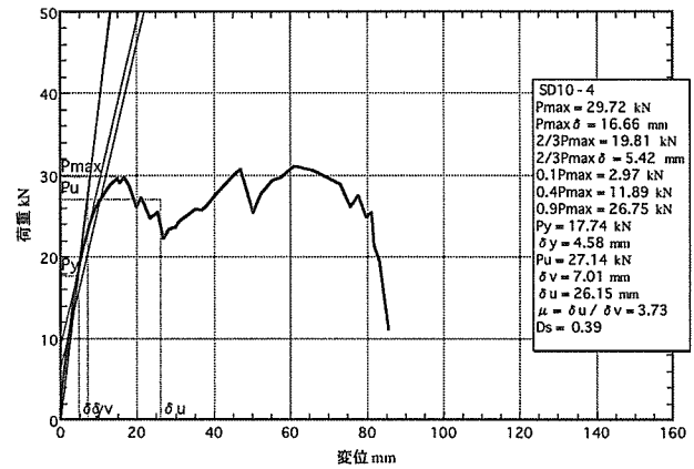
図5. 4 : SD10-4の荷重-変位包絡線
