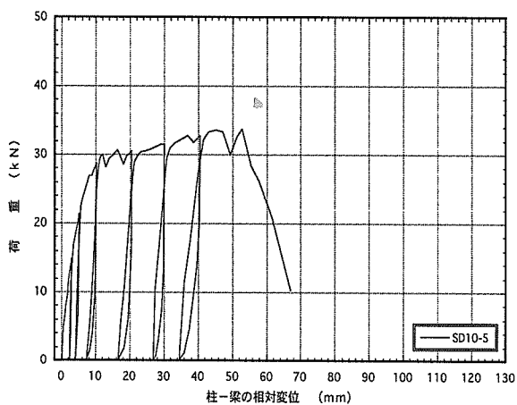
図4. 5 : SD10-5 梁受け金物DB-10のせん断荷試験の荷重-変位曲線
