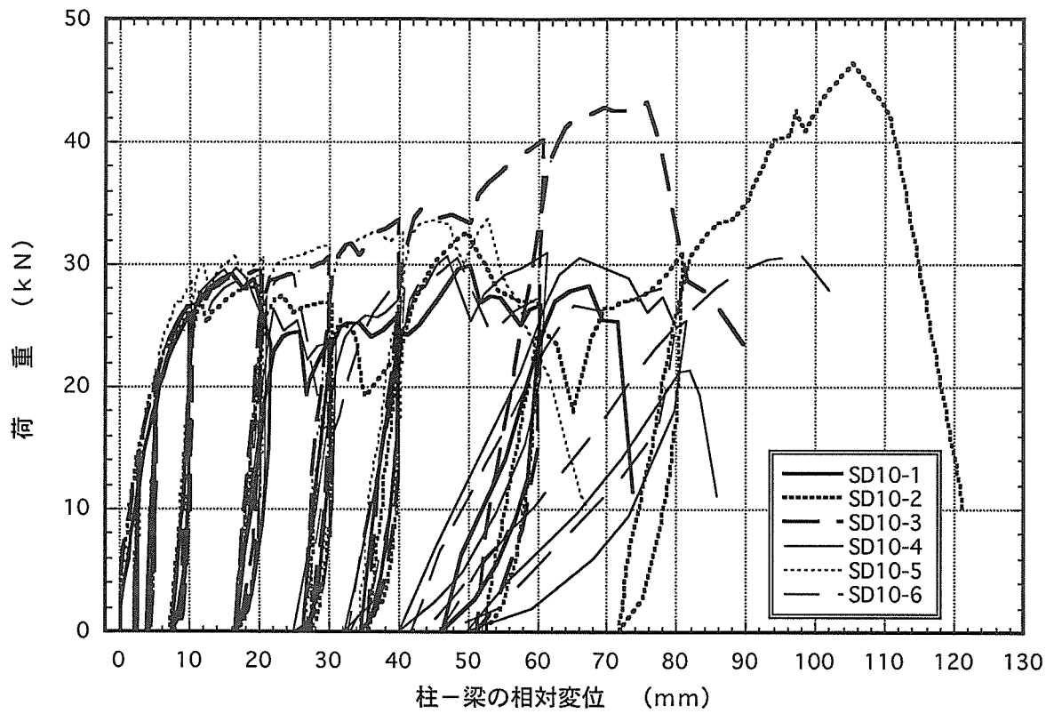
図4. 7 : SD10 梁受け金物DB-10のせん断載荷試験の荷重-変位曲線
