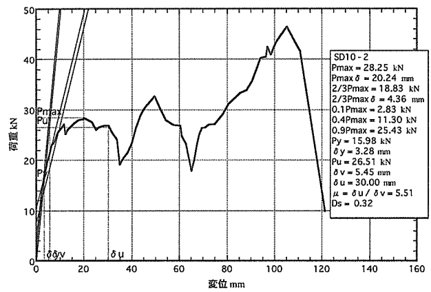
図5. 2 : SD10-2の荷重-変位包絡線
