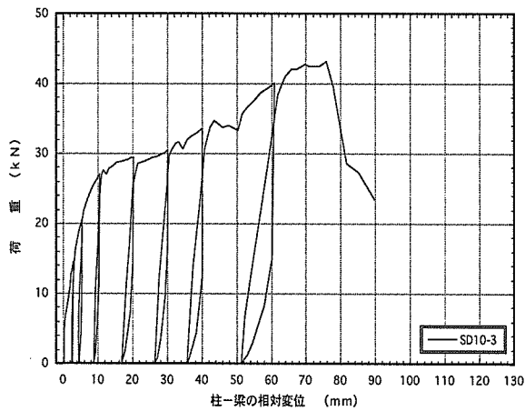
図4. 3 : SD10-3 梁受け金物DB-10のせん断荷試験の荷重-変位曲線
