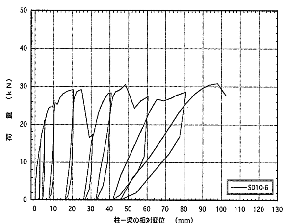
図4. 6 : SD10-6 梁受け金物DB-10のせん断荷試験の荷重-変位曲線
