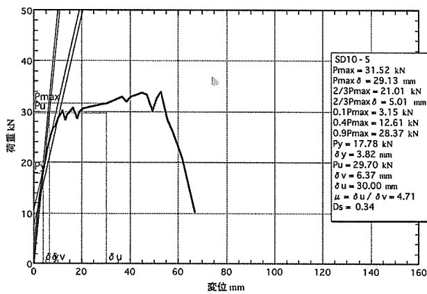
図5. 5 : SD10-5の荷重-変位包絡線
