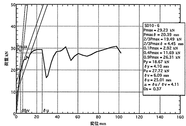
図5. 6 : SD10-6の荷重-変位包絡線
