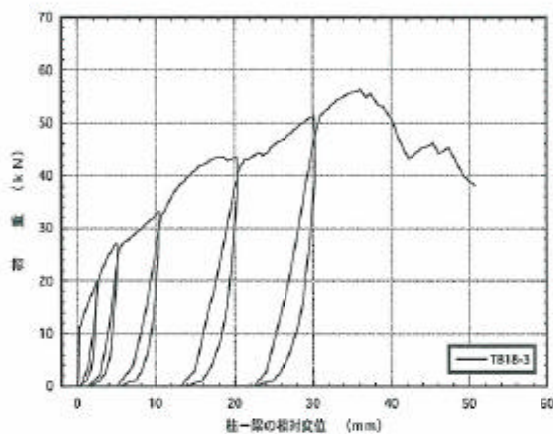
図4. 3 : TB18-3 梁受け金物DB-18の引張載荷試験の荷重-変位曲線
