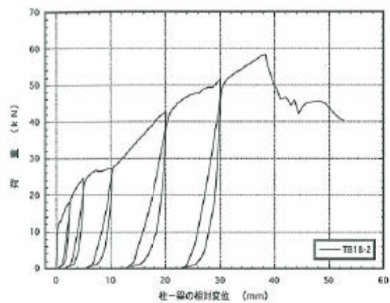
図4. 2 : TB18-2 梁受け金物DB-18の引張載荷試験の荷重-変位曲線
