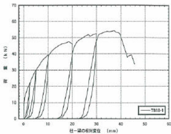
図4. 1 : TB18-1 梁受け金物DB-18の引張載荷試験の荷重-変位曲線
