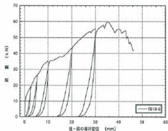
図4. 6 : TB18-6 梁受け金物DB-18の引張載荷試験の荷重-変位曲線
