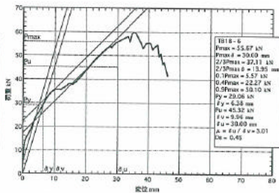
図5.6: TB18-6の荷重-変位包絡線
