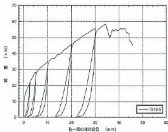
図4. 5 : TB18-5 梁受け金物DB-18の引張載荷試験の荷重-変位曲線
