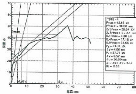
図5.4: TB18-4の荷重-変位包絡線
