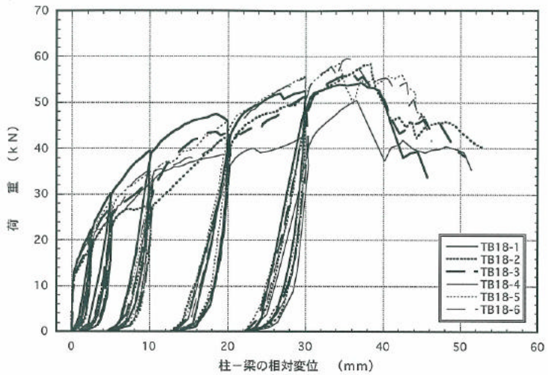
図4. 7 : TB18 梁受け金物DB-18の引張載荷試験の荷重-変位曲線
