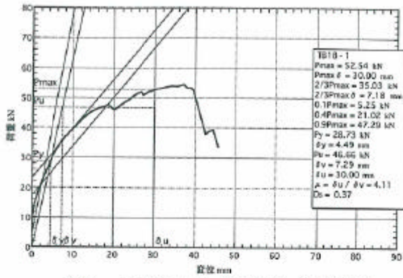
図5.1: TB18-1の荷重-変位包絡線
