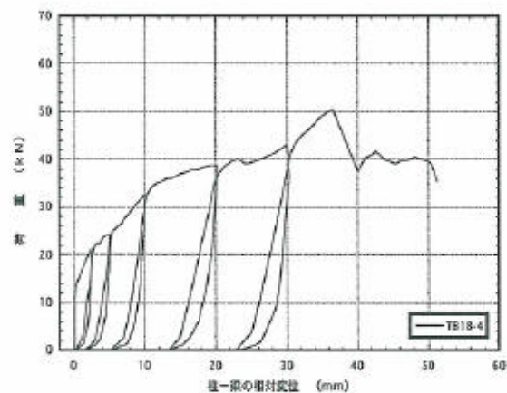
図4. 4 : TB18-4 梁受け金物DB-18の引張載荷試験の荷重-変位曲線
