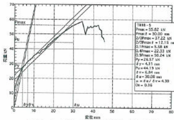
図5.5: TB18-5の荷重-変位包絡線
