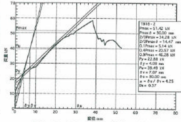
図5.2: TB18-2の荷重-変位包絡線
