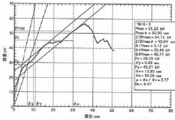
図5.3: TB18-3の荷重-変位包絡線
