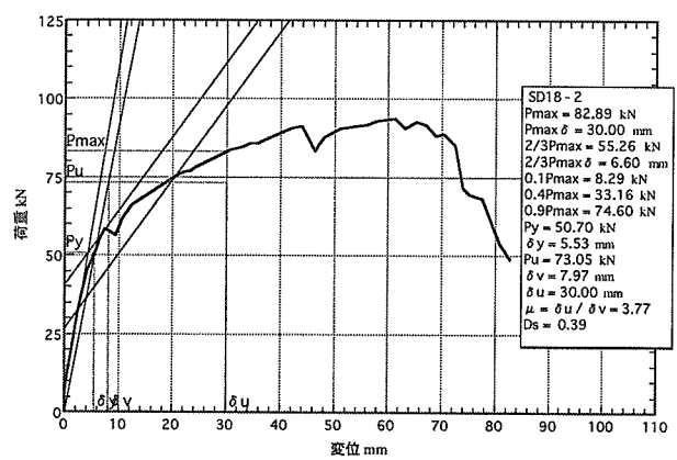
図 5. 2 : SD18-2 の荷重-変位包絡線
