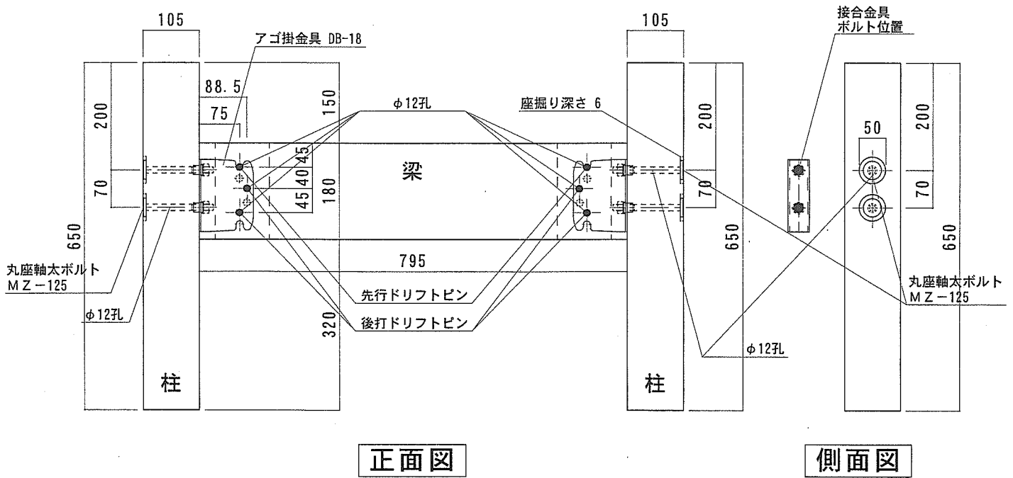
上面図
