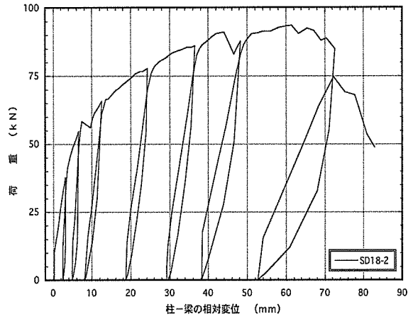
図4. 2 : SD18-2 梁受け金物DB-18のせん断荷試験の荷重-変位曲線
