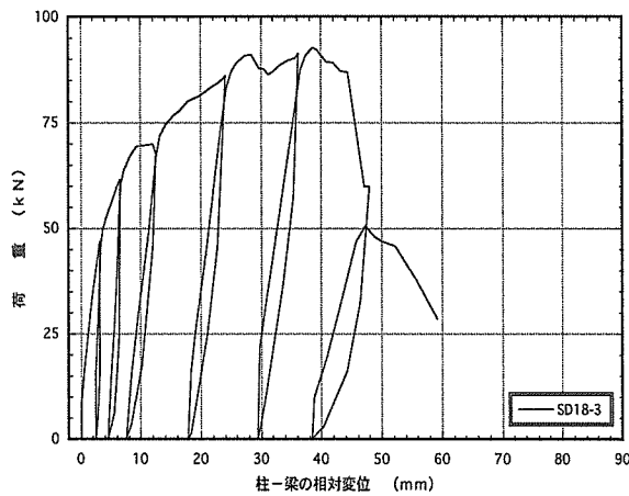
図4. 3 : SD18-3 梁受け金物DB-18のせん断荷試験の荷重-変位曲線
