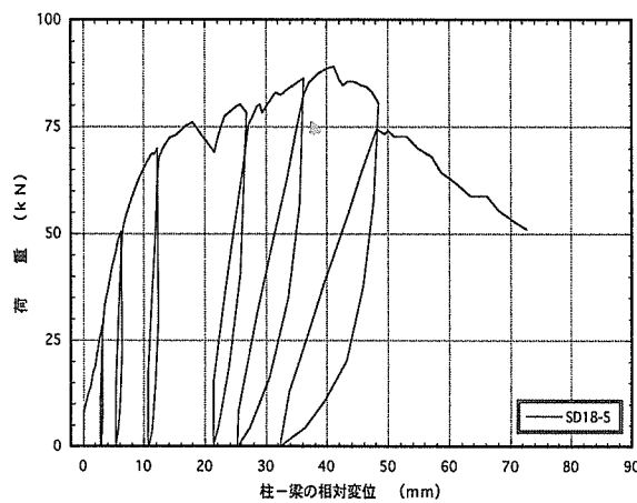
図4. 5 : SD18-5 梁受け金物DB-18のせん断荷試験の荷重-変位曲線
