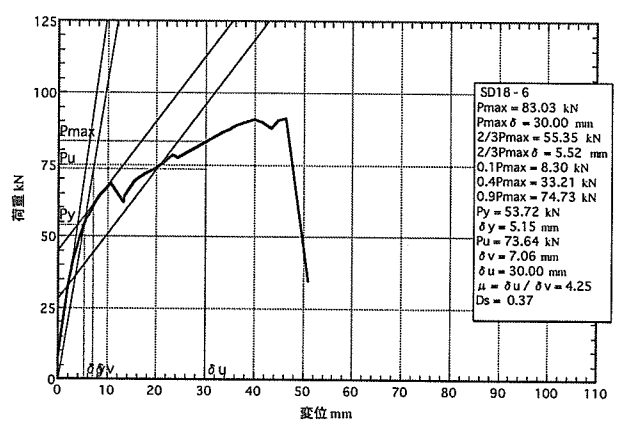
図 5. 6 : SD18-6 の荷重-変位包絡線
