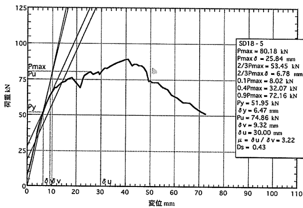
図 5. 5 : SD18-5 の荷重-変位包絡線
