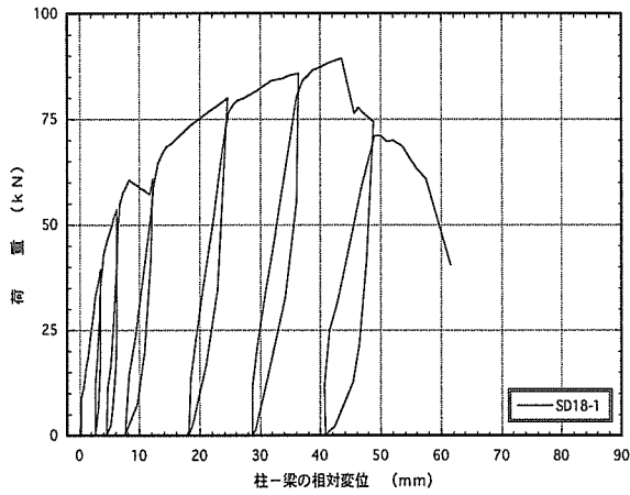
図4. 1 : SD18-1 梁受け金物DB-18のせん断荷試験の荷重-変位曲線
