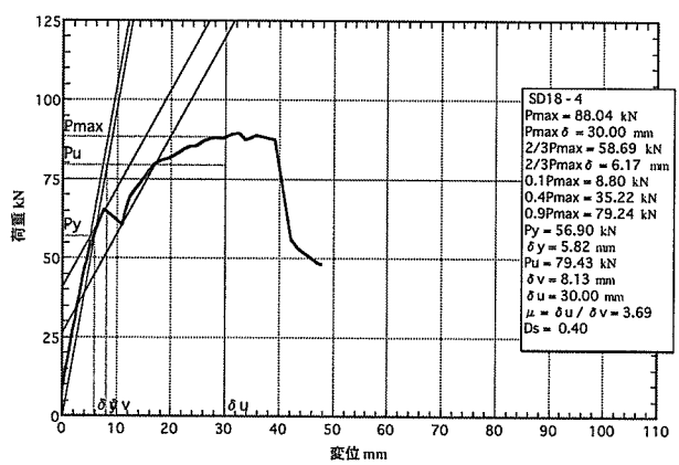
図 5. 4 : SD18-4 の荷重-変位包絡線
