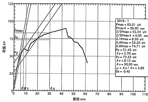
図 5. 1 : SD18-1 の荷重-変位包絡線
