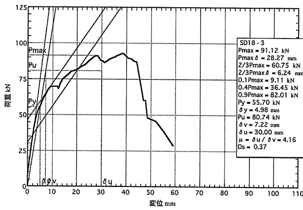
図 5. 3 : SD18-3 の荷重-変位包絡線
