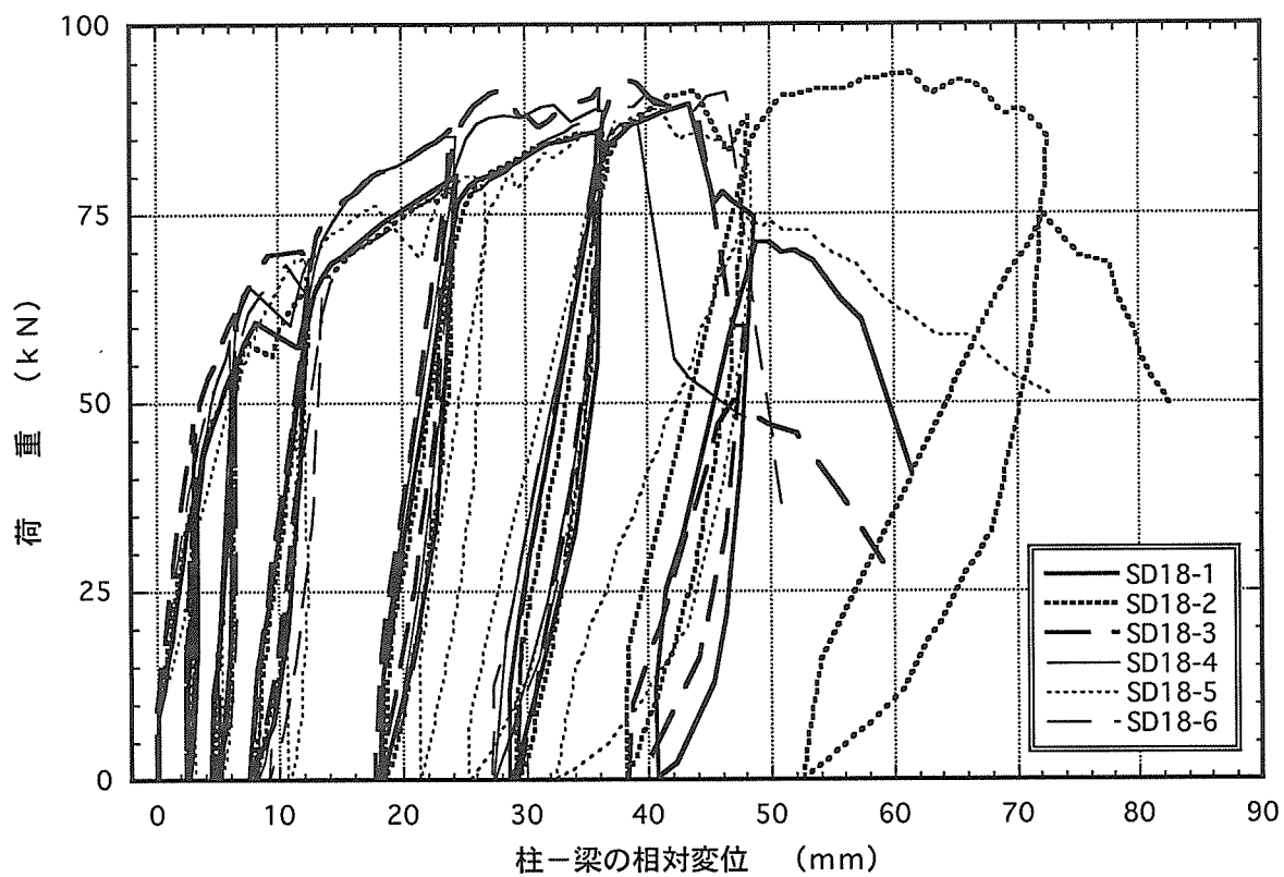
図4. 7 : SD18 梁受け金物DB-18のせん断載荷試験の荷重-変位曲線
