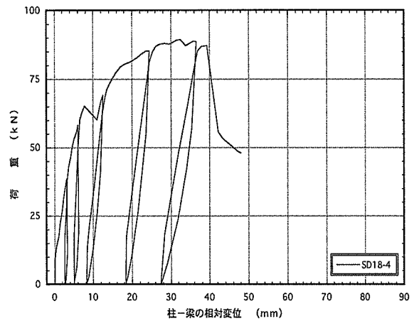
図4. 4 : SD18-4 梁受け金物DB-18のせん断荷試験の荷重-変位曲線
