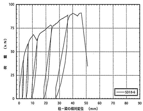
図4. 6 : SD18-6 梁受け金物DB-18のせん断荷試験の荷重-変位曲線
