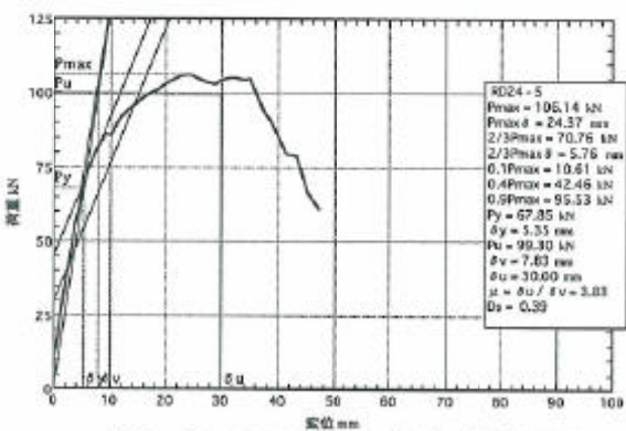
図5.5: RD24-5の荷重-変位包絡線
