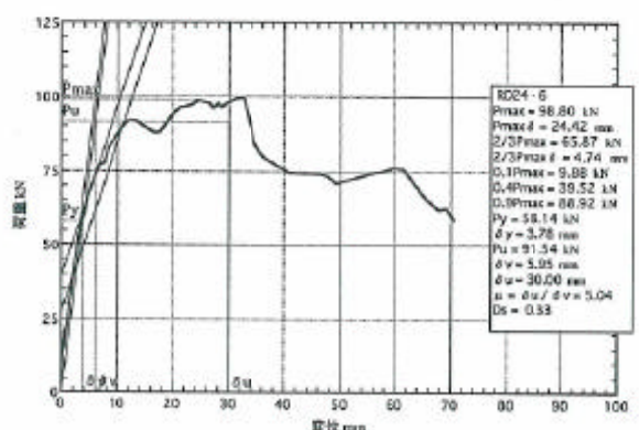
図5.6: RD24-6の荷重-変位包絡線
