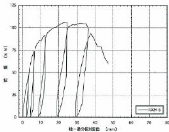
図4. 5 : RD24-5 梁受け金物DB-24の逆せん断載荷試験の荷重-変位曲線
