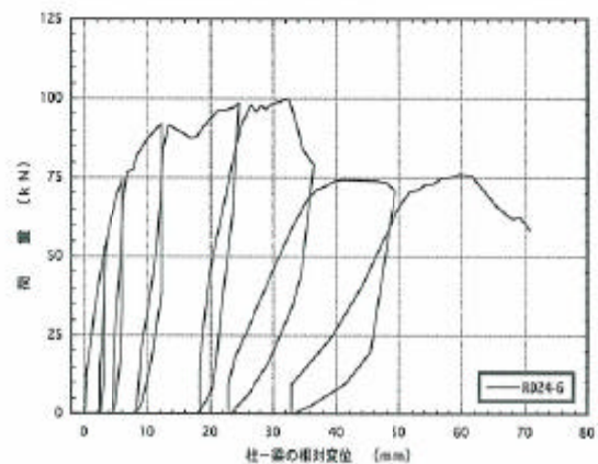
図4. 6 : RD24-6 梁受け金物DB-24の逆せん断載荷試験の荷重-変位曲線
