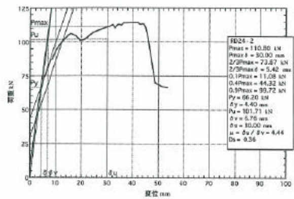
図5.2: RD24-2の荷重-変位包絡線
