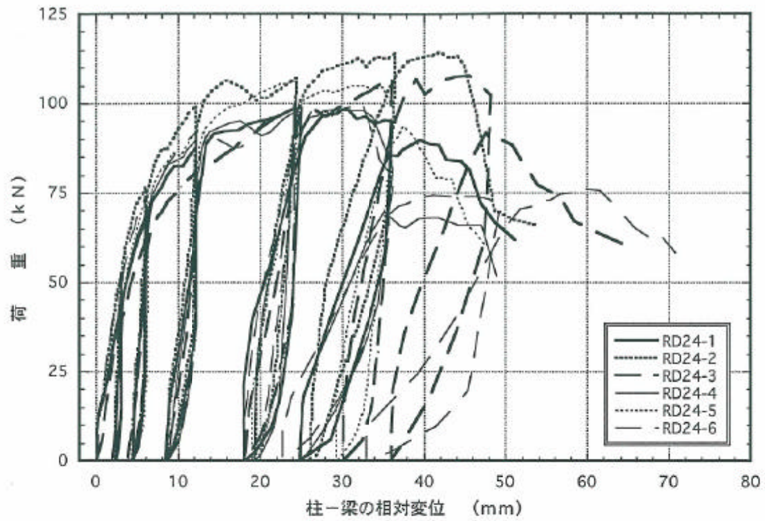
図4. 7 : RD24 梁受け金物DB-24の逆せん断載荷試験の荷重-変位曲線
