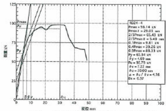
図5.4: RD24-4の荷重-変位包絡線
