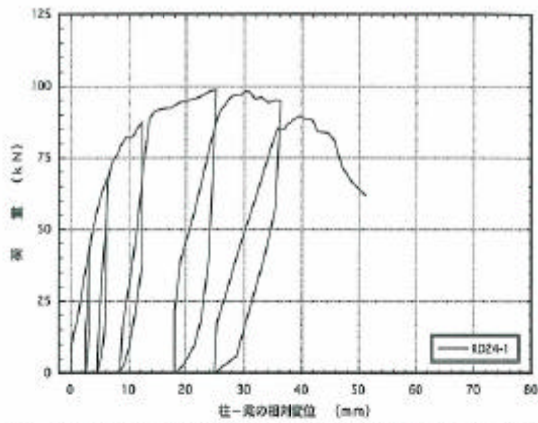
図4. 1 : RD24-1 梁受け金物DB-24の逆せん断載荷試験の荷重-変位曲線
