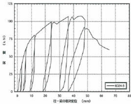
図4. 3 : RD24-3 梁受け金物DB-24の逆せん断載荷試験の荷重-変位曲線
