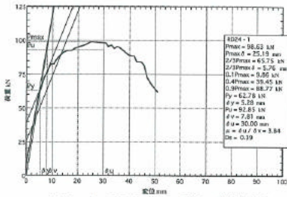
図5.1: RD24-1の荷重-変位包絡線
