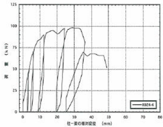
図4. 4 : RD24-4 梁受け金物DB-24の逆せん断載荷試験の荷重-変位曲線
