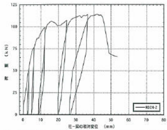
図4. 2 : RD24-2 梁受け金物DB-24の逆せん断載荷試験の荷重-変位曲線
