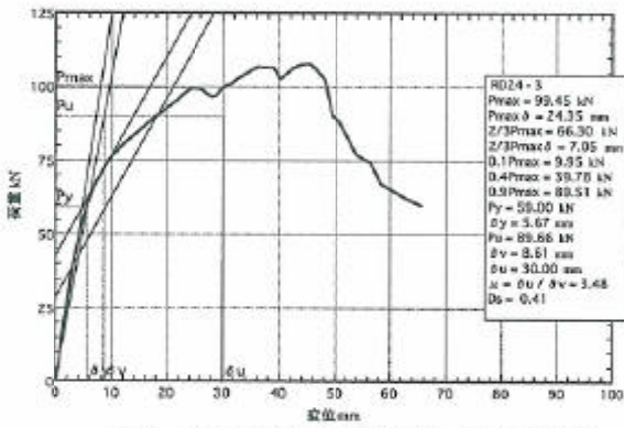
図5.3: RD24-3の荷重-変位包絡線
