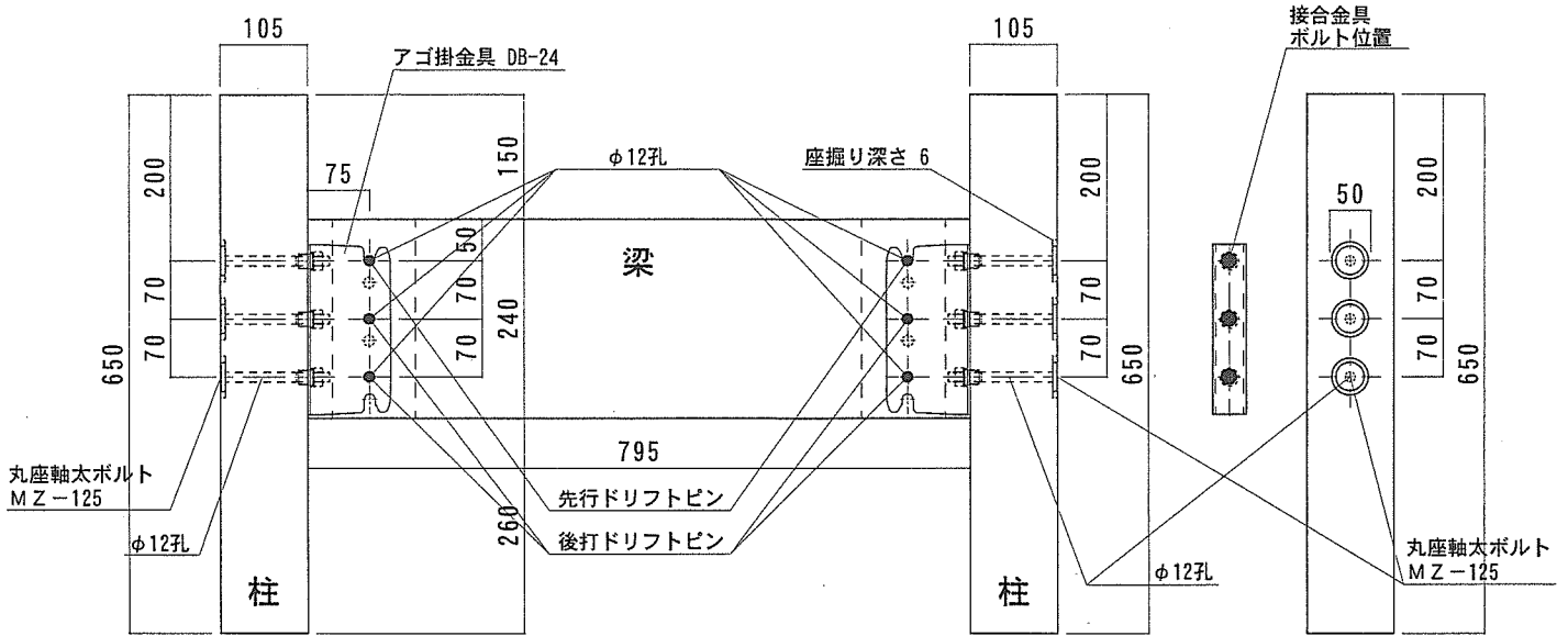
正面図
