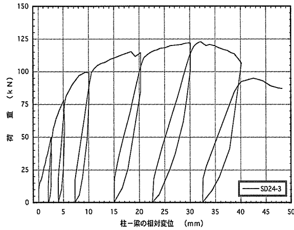
図4. 3 : SD24-3 梁受け金物DB-24のせん断荷試験の荷重-変位曲線
