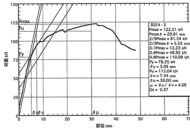
図5. 3 : SD24-3の荷重-変位包絡線
