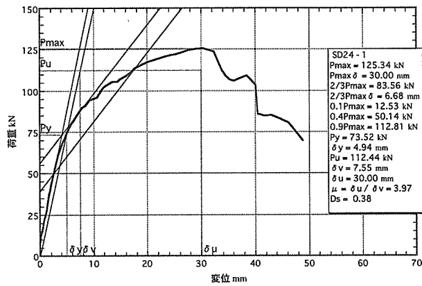
図5. 1 : SD24-1の荷重-変位包絡線
