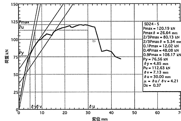
図5. 5 : SD24-5の荷重-変位包絡線
