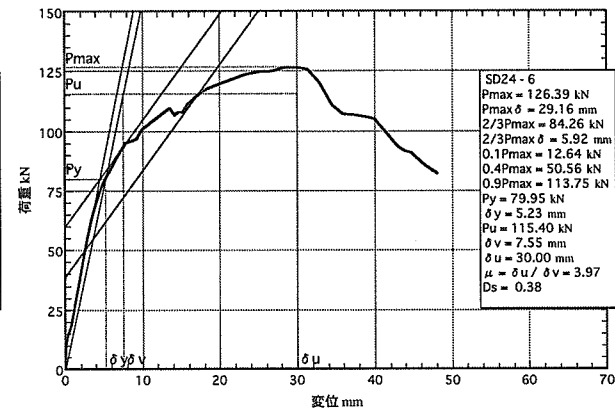
図5. 6 : SD24-6の荷重-変位包絡線
