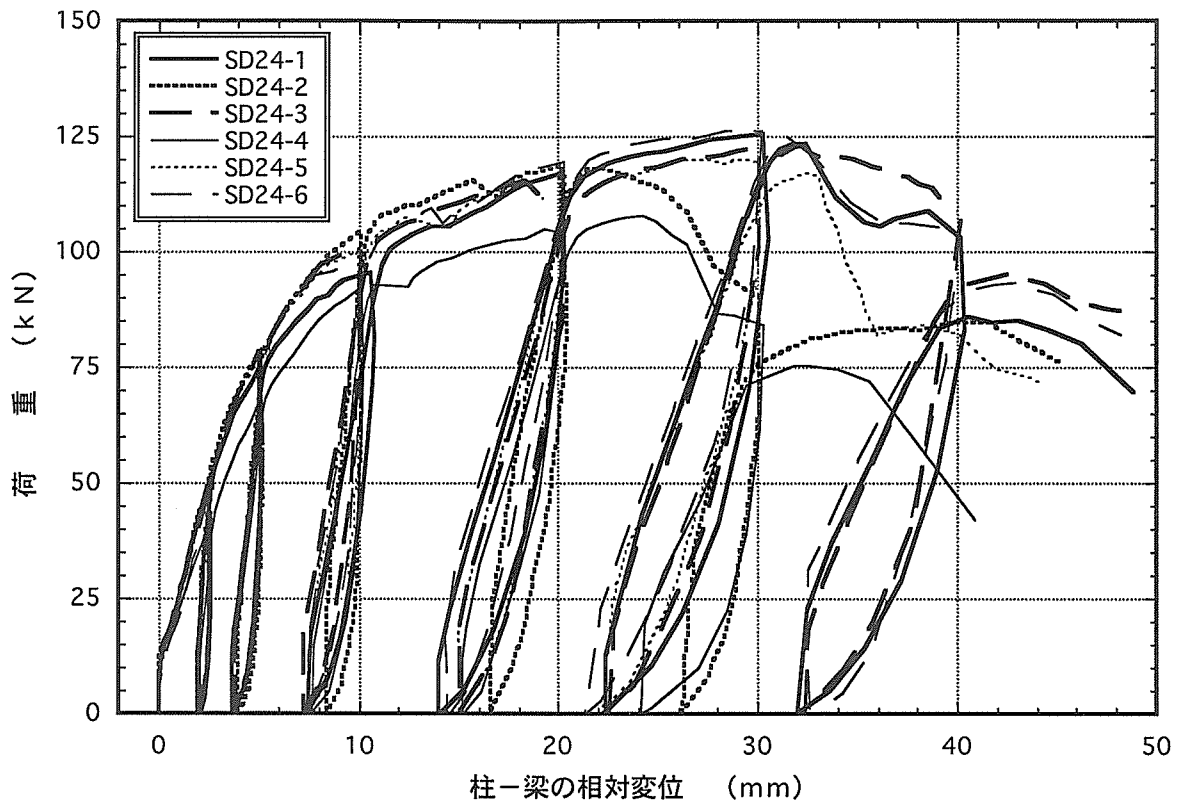
図4. 7 : SD24 梁受け金物DB-24のせん断載荷試験の荷重-変位曲線
