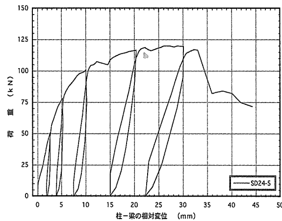
図4. 5 : SD24-5 梁受け金物DB-24のせん断荷試験の荷重-変位曲線
