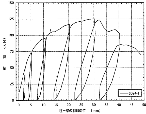
図4. 1 : SD24-1 梁受け金物DB-24のせん断荷試験の荷重-変位曲線
