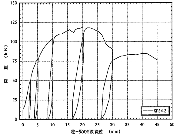
図4. 2 : SD24-2 梁受け金物DB-24のせん断荷試験の荷重-変位曲線
