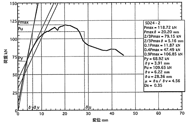
図5. 2 : SD24-2の荷重-変位包絡線
