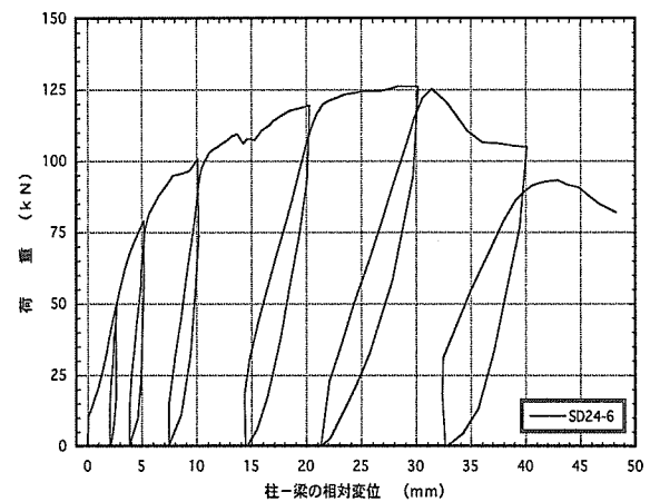
図4. 6 : SD24-6 梁受け金物DB-24のせん断荷試験の荷重-変位曲線
