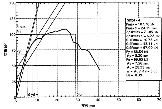
図5. 4 : SD24-4の荷重-変位包絡線
