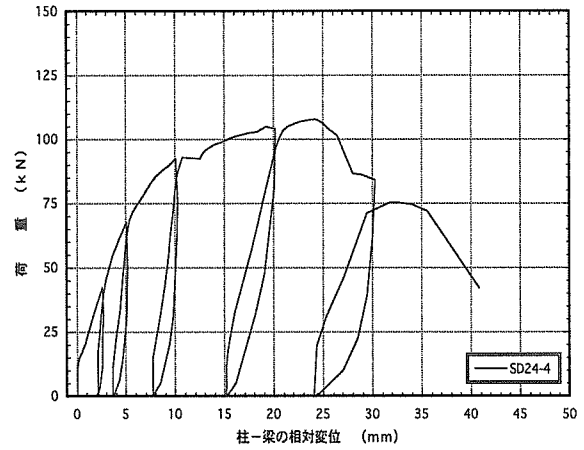
図4. 4 : SD24-4 梁受け金物DB-24のせん断荷試験の荷重-変位曲線
