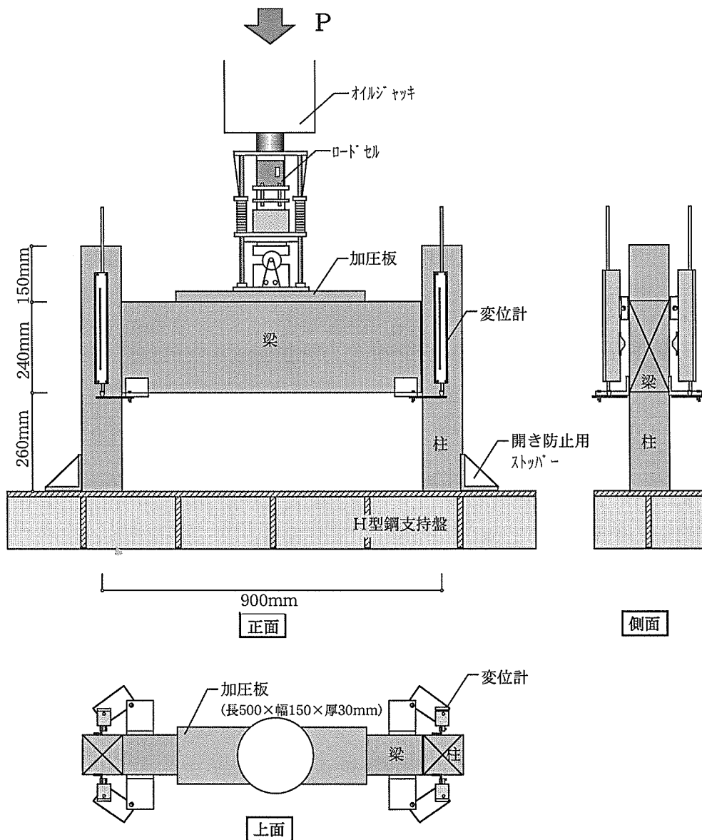
図3. 1：柱－梁接合部の圧縮型せん断载荷試験方法
