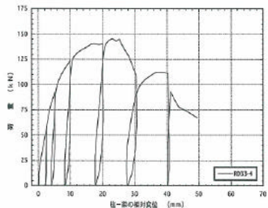
図4. 4 : RD33-4 梁受け金物DB-33の逆せん断荷試験の荷重-変位曲線
