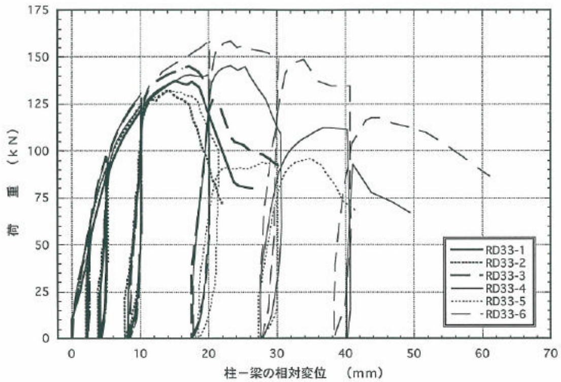
図4. 7 : RD33 梁受け金物DB-33の逆せん断載荷試験の荷重-変位曲線
