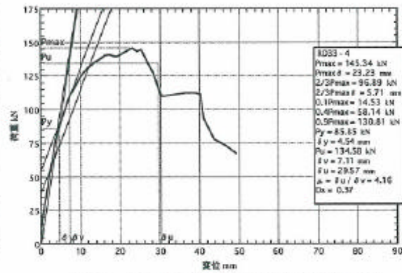
図5. 4 : RD33-4の荷重-変位包絡線
