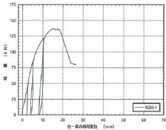
図4. 1 : RD33-1 梁受け金物DB-33の逆せん断荷試験の荷重-変位曲線
