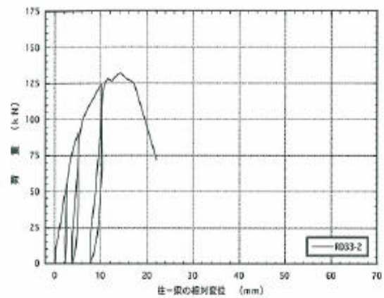
図4. 2 : RD33-2 梁受け金物DB-33の逆せん断荷試験の荷重-変位曲線
