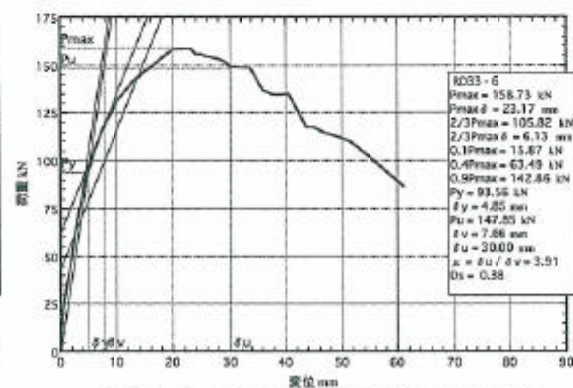
図5. 6 : RD33-6の荷重-変位包絡線
