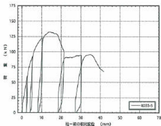
図4. 5 : RD33-5 梁受け金物DB-33の逆せん断荷試験の荷重-変位曲線
