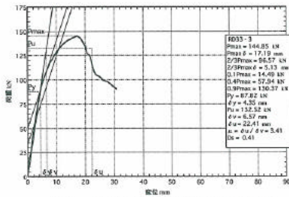
図5. 3 : RD33-3の荷重-変位包絡線
