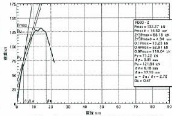
図5. 2 : RD33-2の荷重-変位包絡線
