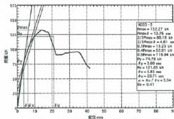
図5. 5 : RD33-5の荷重-変位包絡線
