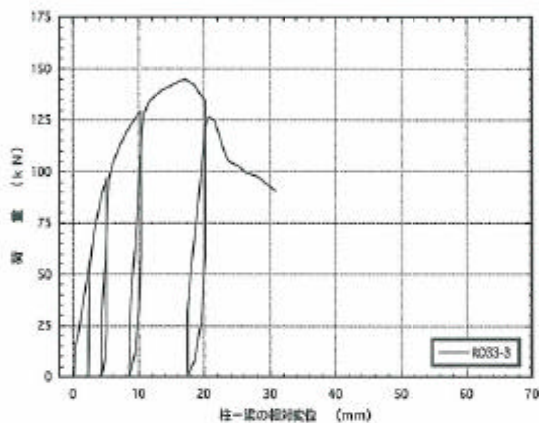
図4. 3 : RD33-3 梁受け金物DB-33の逆せん断荷試験の荷重-変位曲線
