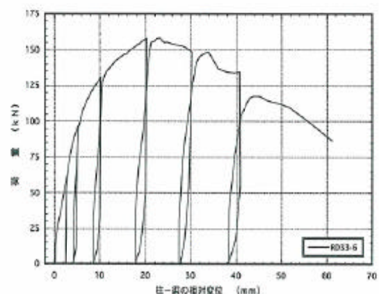
図4. 6 : RD33-6 梁受け金物DB-33の逆せん断荷試験の荷重-変位曲線
