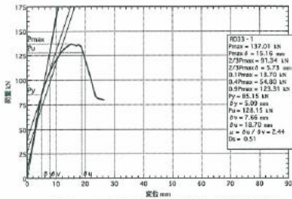
図5. 1 : RD33-1の荷重-変位包絡線
