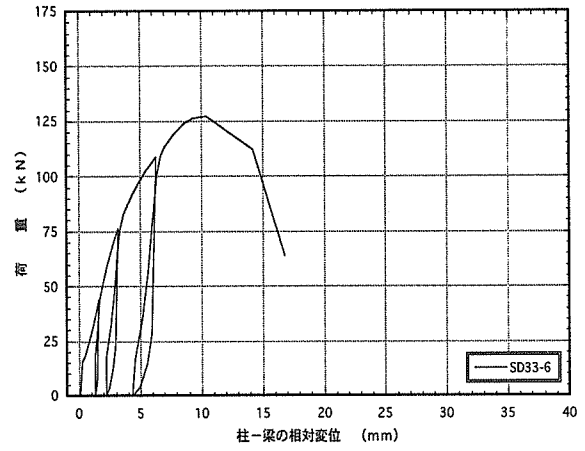
図4. 6 : SD33-6 梁受け金物DB-33のせん断荷試験の荷重-変位曲線
