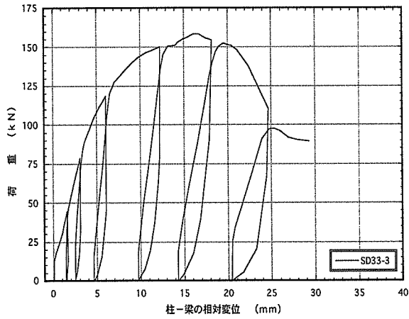
図4. 3 : SD33-3 梁受け金物DB-33のせん断荷試験の荷重-変位曲線
