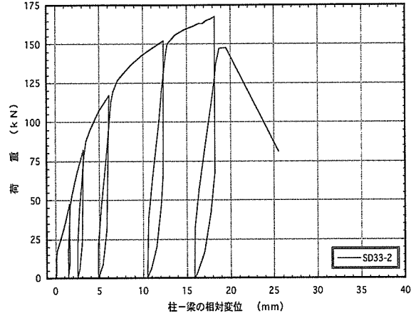
図4. 2 : SD33-2 梁受け金物DB-33のせん断荷試験の荷重-変位曲線
