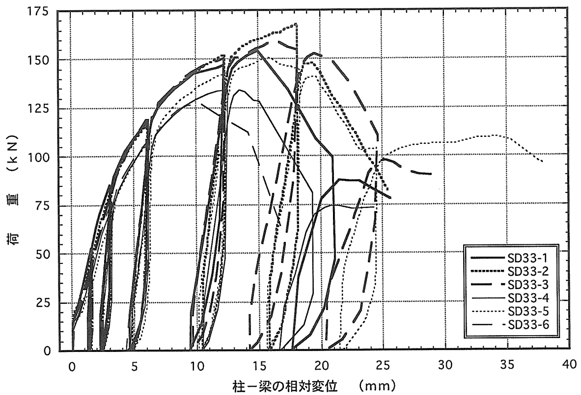
図4. 7 : SD33 梁受け金物DB-33のせん断載荷試験の荷重-変位曲線
