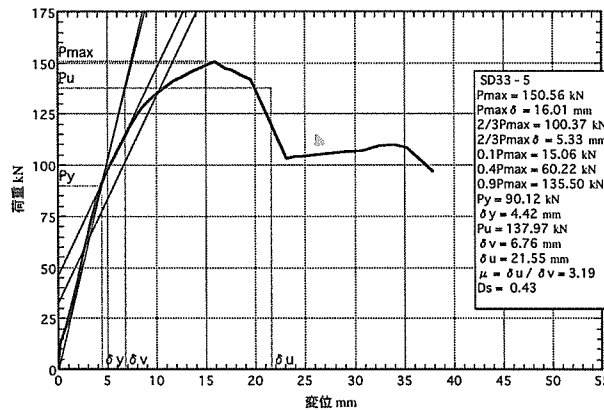
図5. 5 : SD33-5の荷重-変位包絡線
