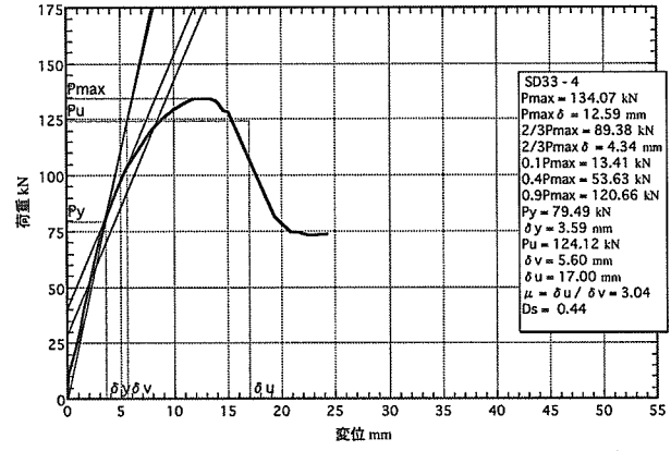
図5. 4 : SD33-4の荷重-変位包絡線
