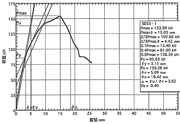
図5. 1 : SD33-1の荷重-変位包絡線
