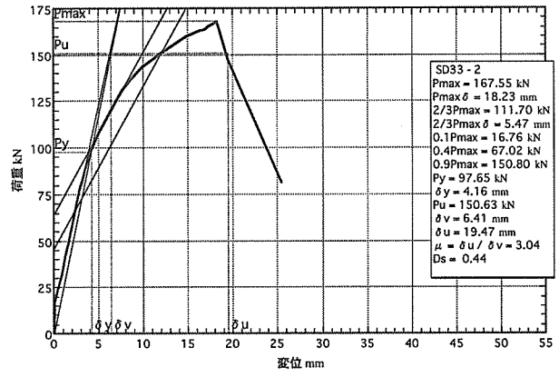
図5. 2 : SD33-2の荷重-変位包絡線
