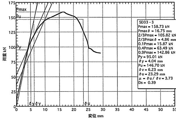
図5. 3 : SD33-3の荷重-変位包絡線
