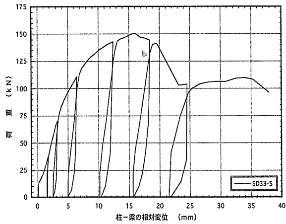
図4. 5 : SD33-5 梁受け金物DB-33のせん断荷試験の荷重-変位曲線
