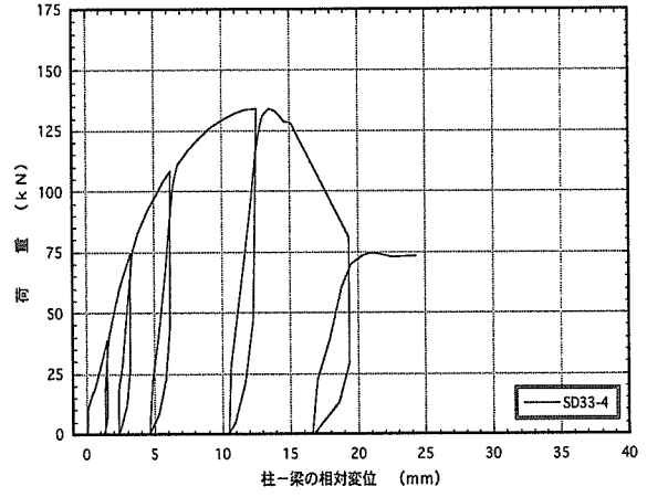
図4. 4 : SD33-4 梁受け金物DB-33のせん断荷試験の荷重-変位曲線
