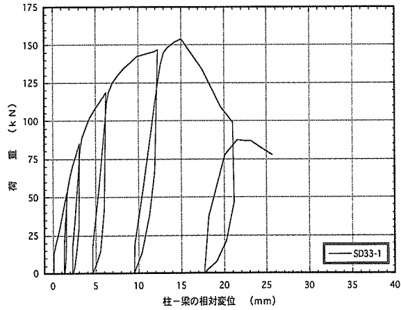
図4. 1 : SD33-1 梁受け金物DB-33のせん断荷試験の荷重-変位曲線
