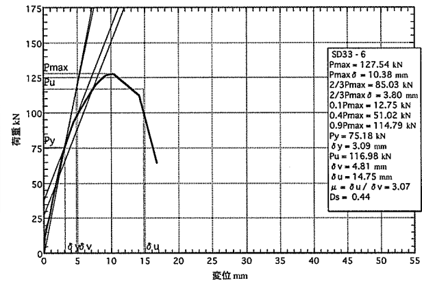
図5. 6 : SD33-6の荷重-変位包絡線
