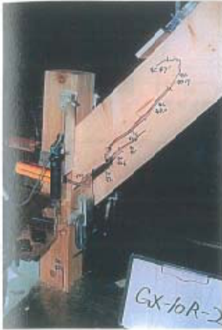
写真-7 破壊状況
