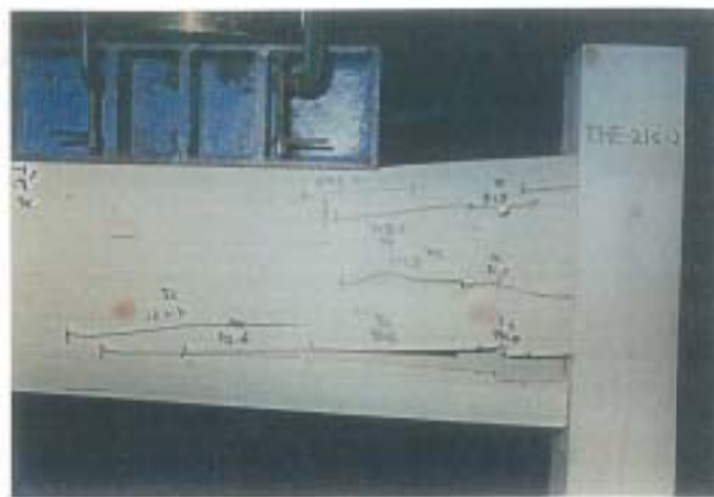
写真-2 破壊状況 試験体記号: THE-215-2 破壊荷重: 60.2kN 30mm 以内の最大荷重: 59.6kN
