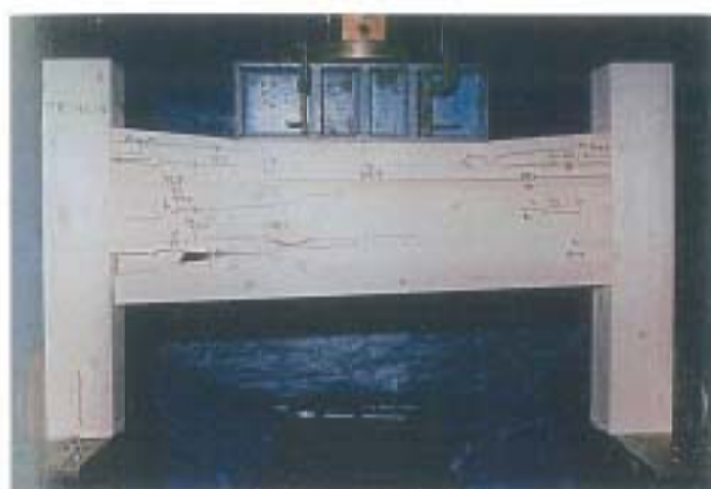
写真-3 破壊状況 試験体記号: THE-215-3 破壊荷重: 59.6kN 30mm 以内の最大荷重: 57.7kN
