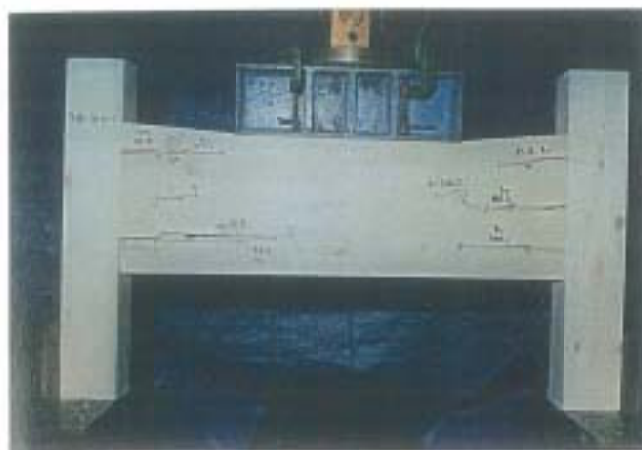
写真-1 破壊状況 試験体記号: THE-215-1 最大荷重: 54.7kN
