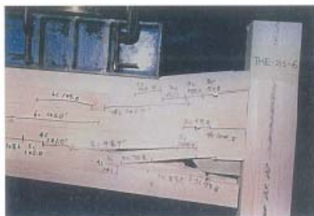
写真-6 破壊状況 試験体記号: THE-215-6 破壊荷重: 54.3kN 30mm 以内の最大荷重: 52.2kN
