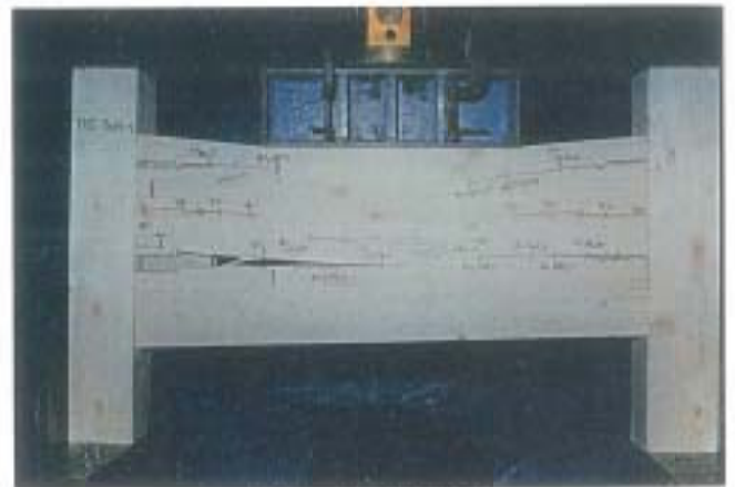
写真-4 破壊状況 試験体記号: THE-30R-4 破壊荷重: 66.8kN 30mm 以内の最大荷重: 65.4kN
