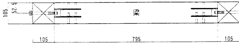
上面図
