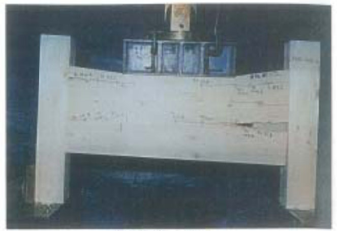
写真-2 破壊状況 試験体記号: THE-30R-2 最大荷重: 60.9kN
