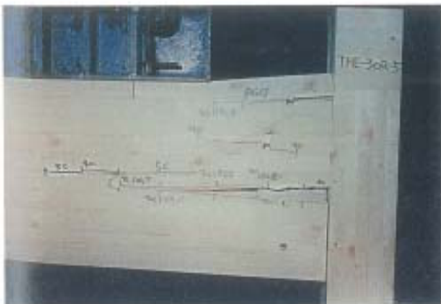
写真-5 破壊状況 試験体記号: THE-30R-5 最大荷重: 64.9kN
