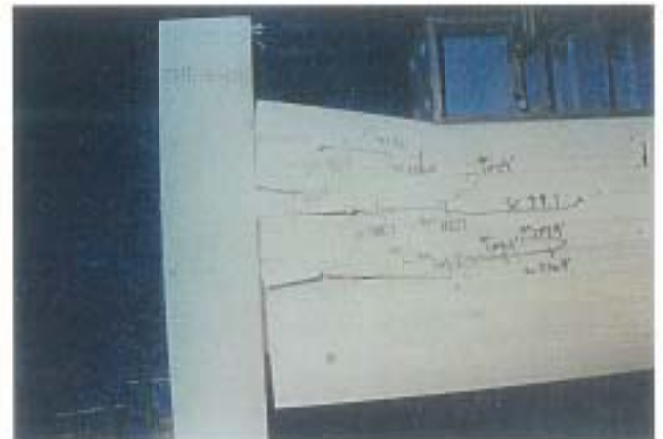
写真-6 破壊状況 試験体記号: THE-30R-6 最大荷重: 64.2kN
