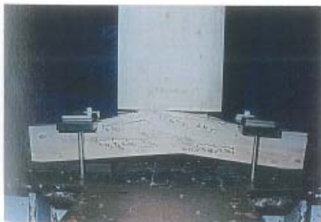
写真-5 破壊状況 試験体記号: THE-30T-5 最大荷重: 85.1kN
