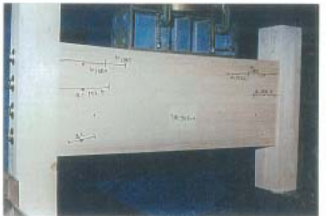
写真-4 破壊状況 試験体記号: THE-30S-4 最大荷重: 77.6kN
