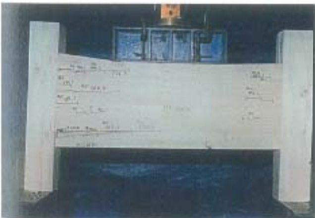
写真-5 破壊状況 試験体記号: THE-30S-5 破壊荷重: 88.7kN 30mm 以内の最大荷重: 87.0kN
