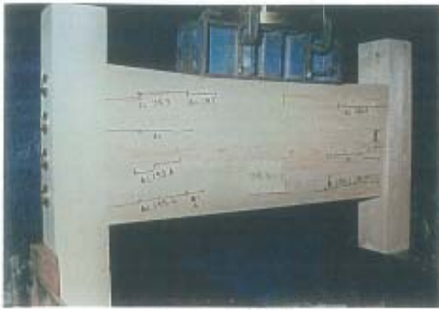
写真-1 破壊状況 試験体記号: THE-30S-1 最大荷重: 78.4kN
