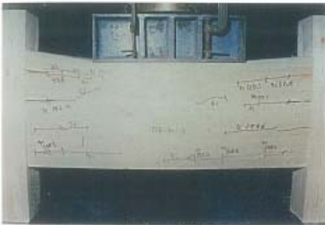
写真-3 破壊状況 試験体記号: THE-30S-3 最大荷重: 89.8kN
