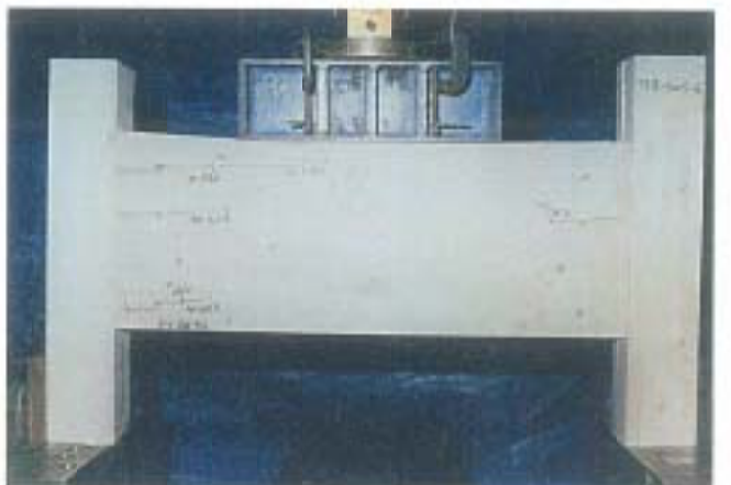
写真-6 破壊状況 試験体記号: THE-30S-6 最大荷重: 77.5kN
