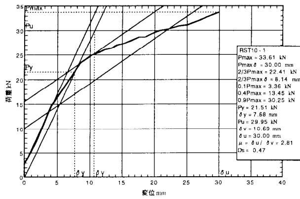
図5. 1 : RST10-1の荷重-変位包絡線
