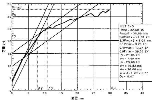
図5. 5 : RST10-5の荷重-変位包絡線
