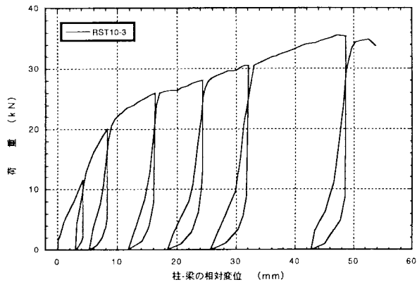
図4. 3:RST10-3 逆付けしたTHF-10のせん断荷試験の荷重-変位曲線
