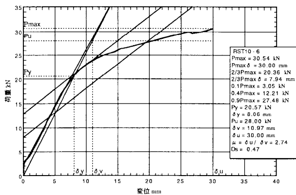
図5. 6 : RST10-6の荷重-変位包絡線
