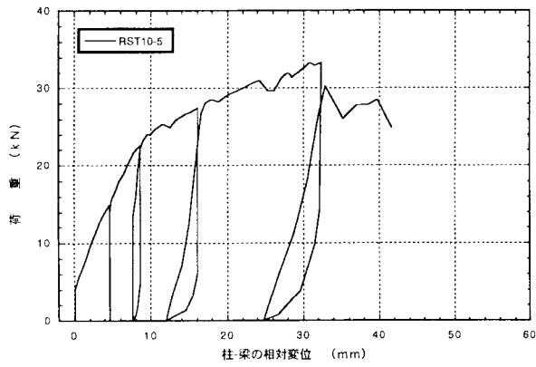
図4. 5:RST10-5 逆付けしたTHF-10のせん断荷試験の荷重-変位曲線
