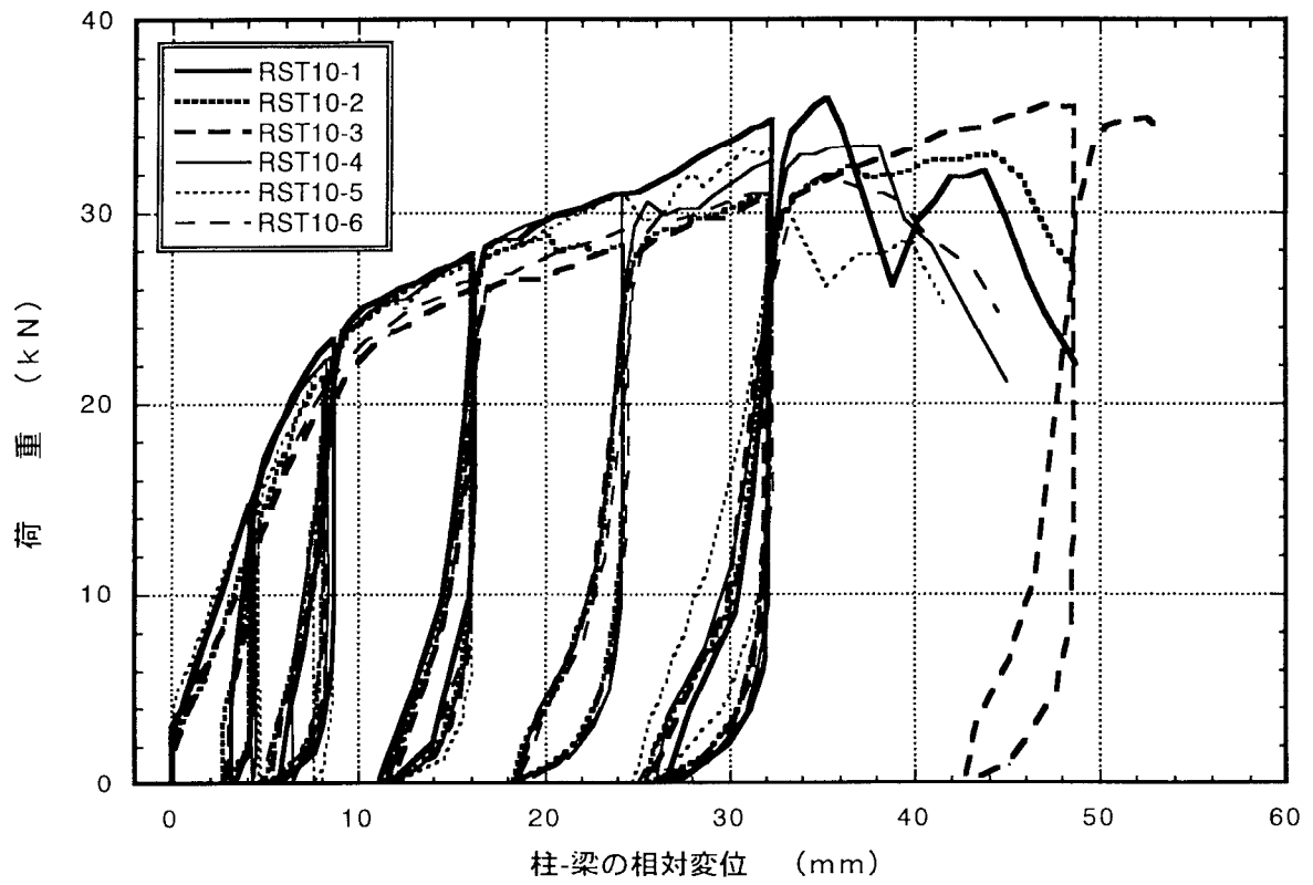
図4. 7:RST10 逆付けしたTHF-10のせん断載荷試験の荷重-変位曲線
