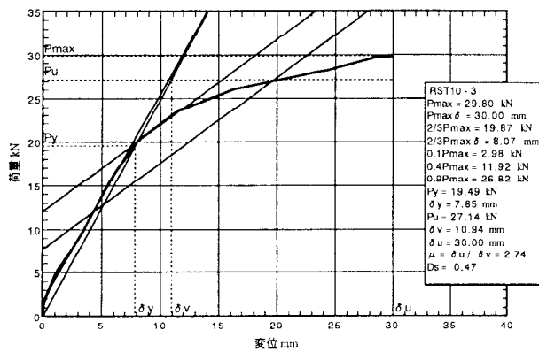
図5. 3 : RST10-3の荷重-変位包絡線
