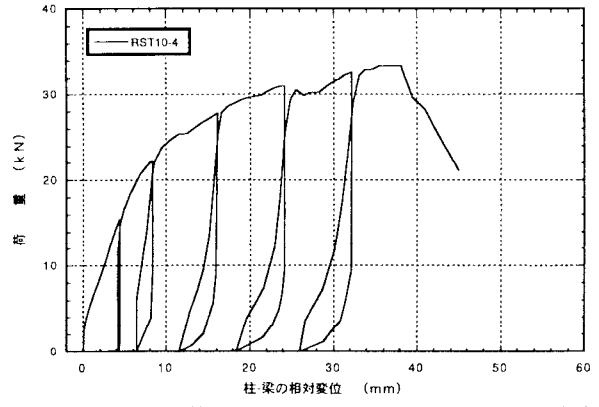
図4. 4:RST10-4 逆付けしたTHF-10のせん断荷試験の荷重-変位曲線
