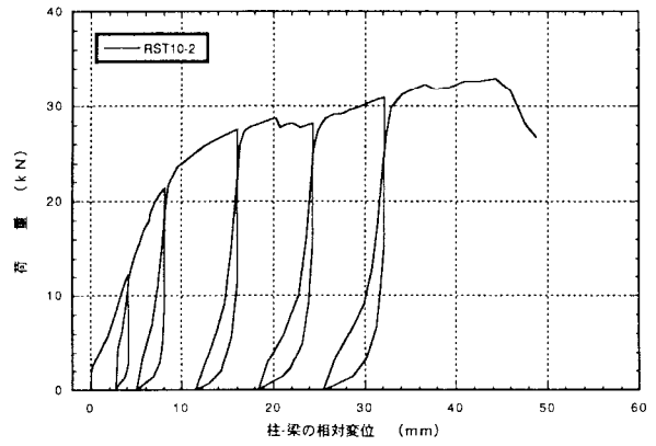
図4. 2:RST10-2 逆付けしたTHF-10のせん断荷試験の荷重-変位曲線
