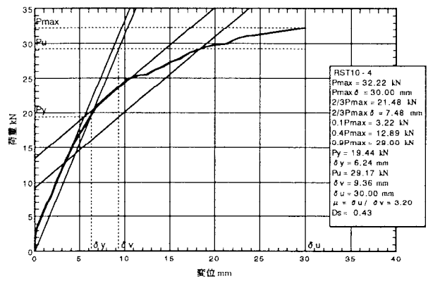
図5. 4 : RST10-4の荷重-変位包絡線
