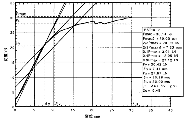
図5. 2 : RST10-2の荷重-変位包絡線
