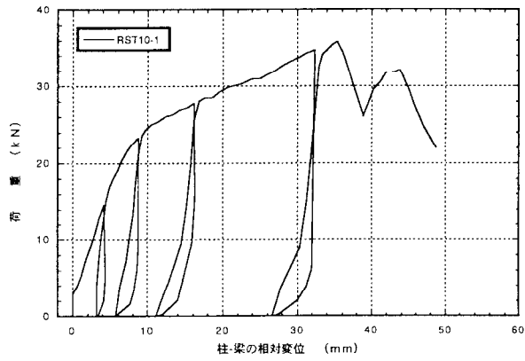
図4. 1:RST10-1 逆付けしたTHF-10のせん断荷試験の荷重-変位曲線
