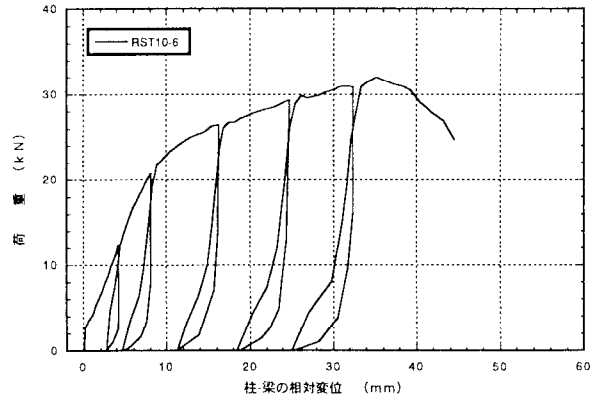
図4. 6:RST10-6 逆付けしたTHF-10のせん断荷試験の荷重-変位曲線
