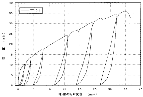
図4. 5 : TT10-5 アゴ掛金物THF-10の引張型荷重試験の荷重-変位曲線
