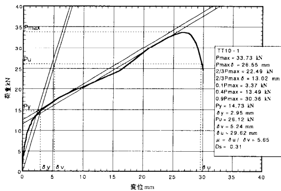
図5. 1 : TT10-1の荷重-変位包絡線
