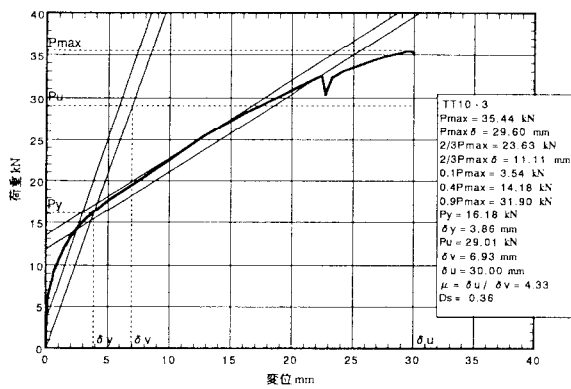
図5. 3 : TT10-3の荷重-変位包絡線
