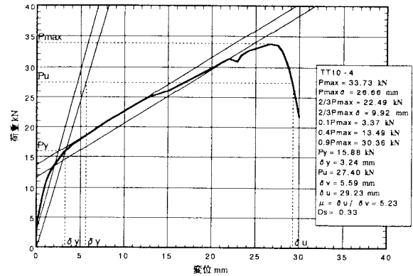
図5. 4 : TT10-4の荷重-変位包絡線
