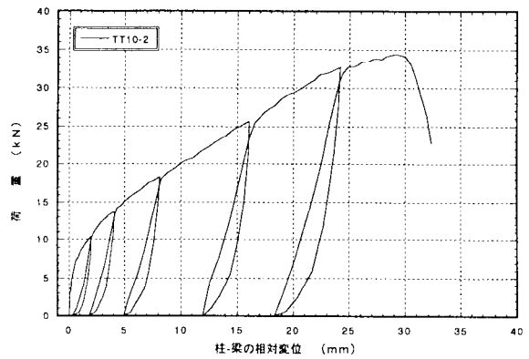
図4. 2 : TT10-2 アゴ掛金物THF-10の引張型荷重試験の荷重-変位曲線
