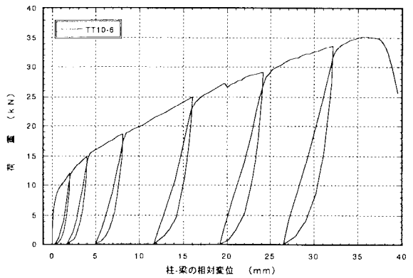
図4. 6 : TT10-6 アゴ掛金物THF-10の引張型荷重試験の荷重-変位曲線
