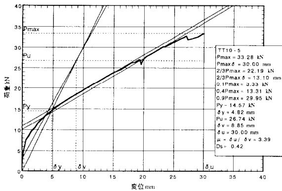
図5. 5 : TT10-5の荷重-変位包絡線
