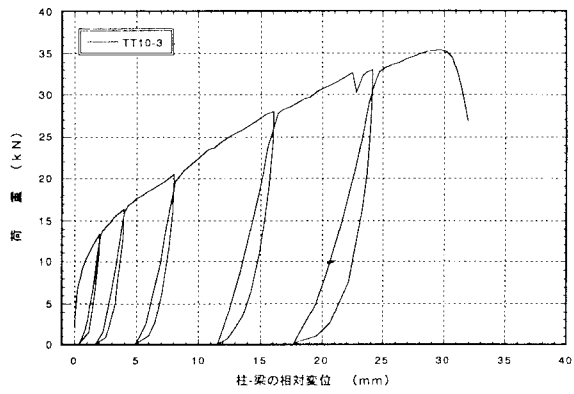
図4. 3 : TT10-3 アゴ掛金物THF-10の引張型荷重試験の荷重-変位曲線
