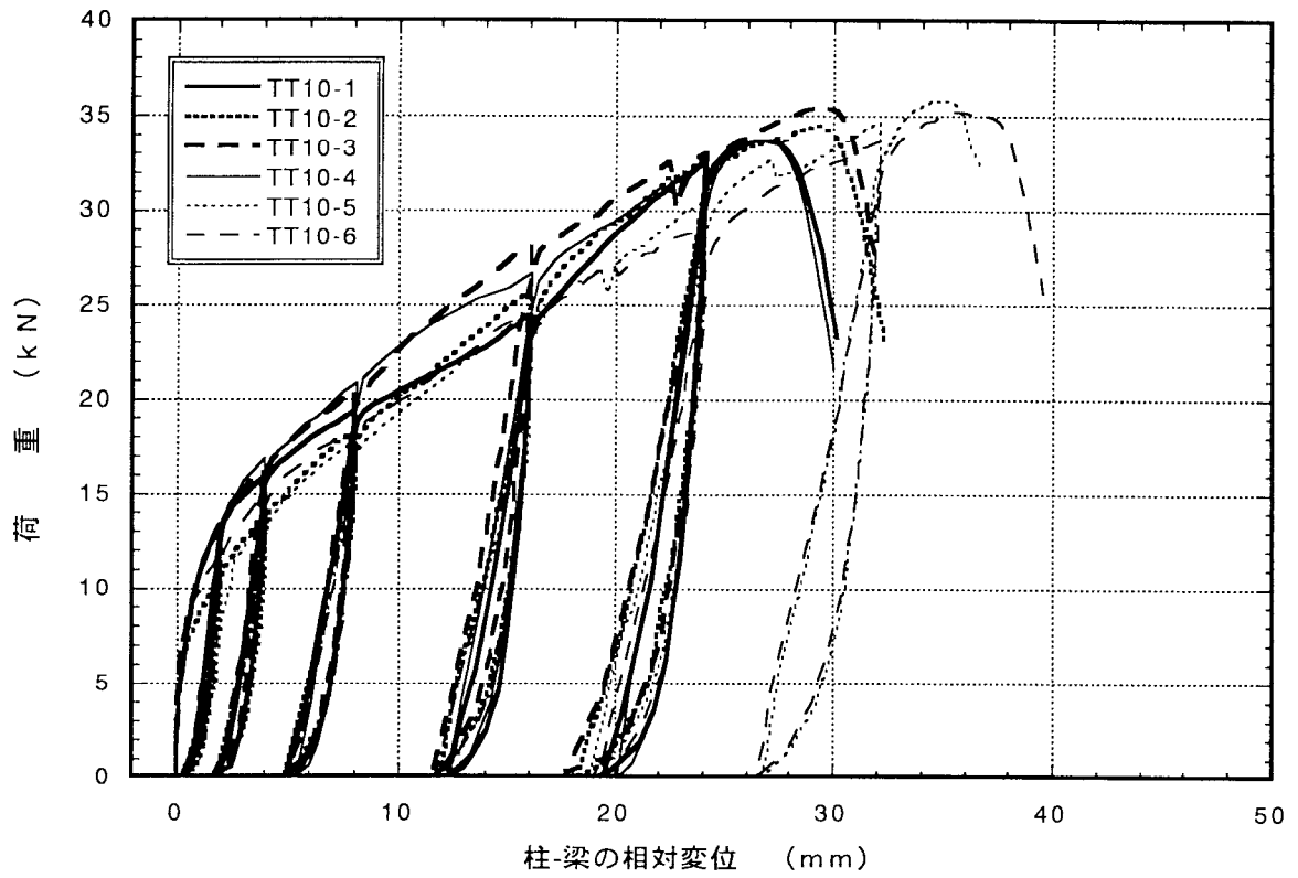
図4. 7 : TT10 アゴ掛金物THF-10の引張型載荷試験の荷重－変位曲線
