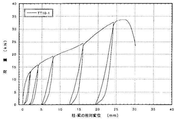
図4. 1 : TT10-1 アゴ掛金物THF-10の引張型荷重試験の荷重-変位曲線
