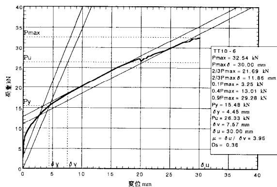
図5. 6 : TT10-6の荷重-変位包絡線
