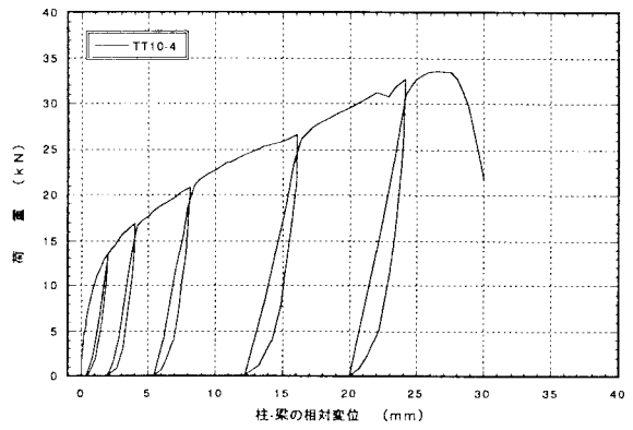
図4. 4 : TT10-4 アゴ掛金物THF-10の引張型荷重試験の荷重-変位曲線
