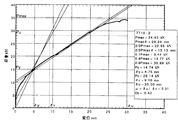
図5. 2 : TT10-2の荷重-変位包絡線
