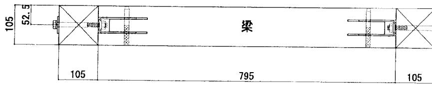
上面図
