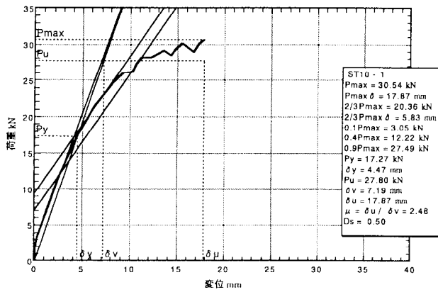
図5. 1 : ST10-1の荷重-変位包絡線
