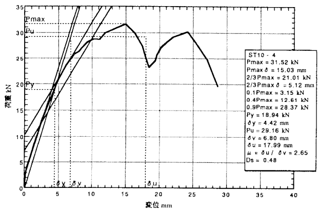
図5. 4 : ST10-4の荷重-変位包絡線
