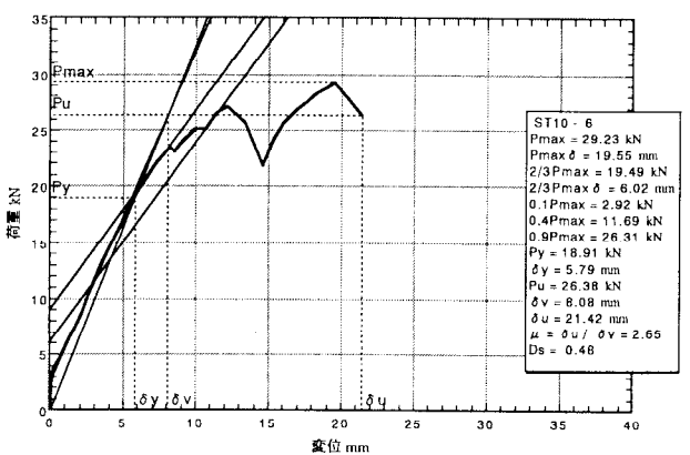
図5. 6 : ST10-6の荷重-変位包絡線
