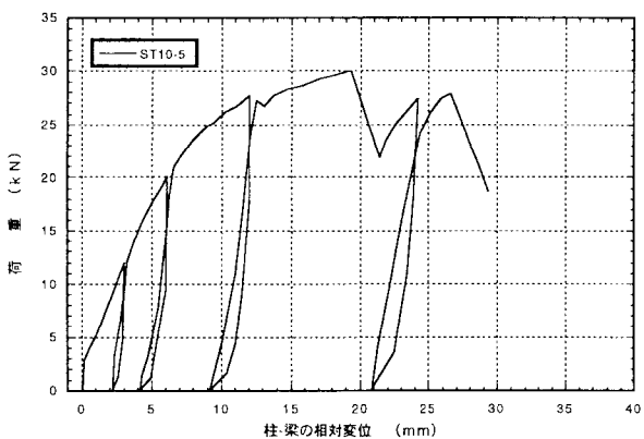
図4. 5 : ST10-5 7' 掛金物THF-10のせん断荷試験の荷重-変位曲線
