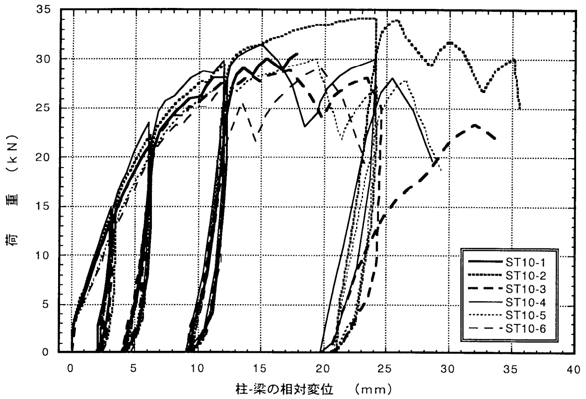
図4. 7 : ST10 7J' 掛金物THF-10のせん断載荷試験の荷重-変位曲線
