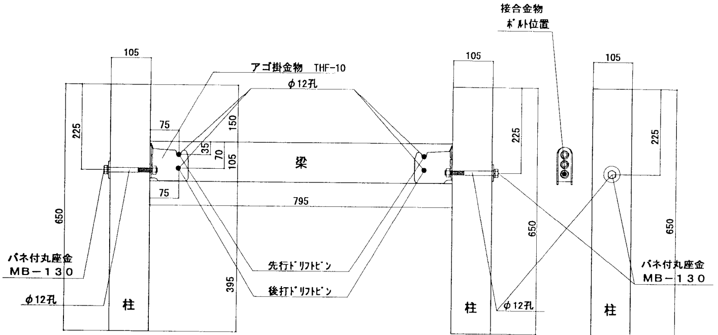
上面図
