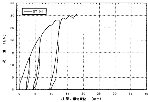
図4. 1 : ST10-1 7' 掛金物THF-10のせん断荷試験の荷重-変位曲線
