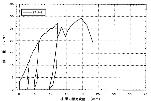
図4. 6 : ST10-6 7' 掛金物THF-10のせん断荷試験の荷重-変位曲線
