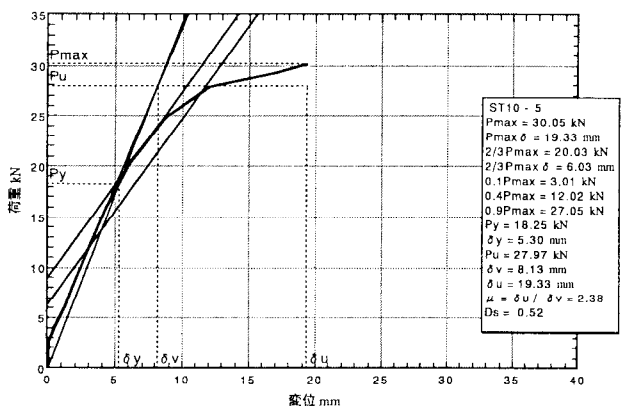
図5. 5 : ST10-5の荷重-変位包絡線
