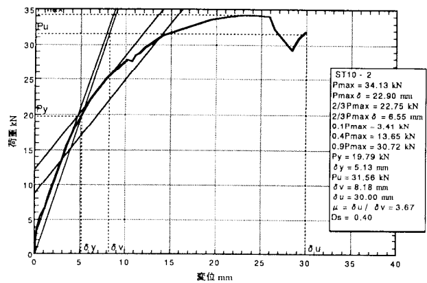
図5. 2 : ST10-2の荷重-変位包絡線
