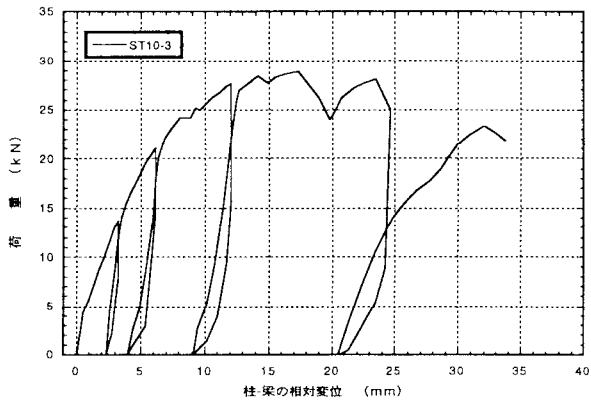
図4. 3 : ST10-3 7' 掛金物THF-10のせん断荷試験の荷重-変位曲線
