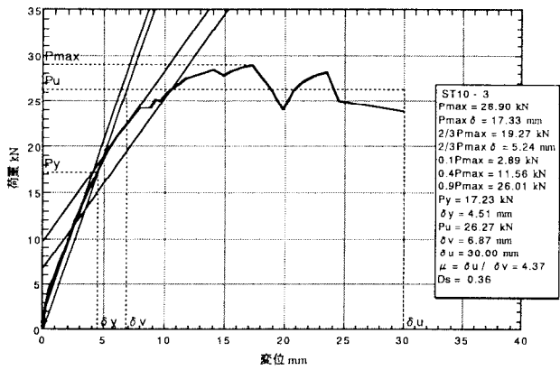
図5. 3 : ST10-3の荷重-変位包絡線
