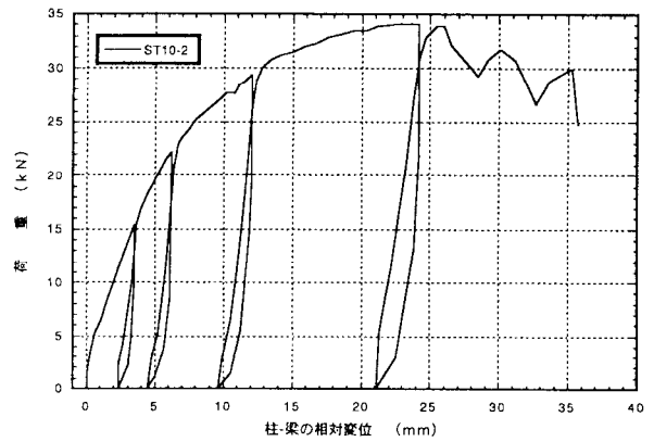
図4. 2 : ST10-2 7' 掛金物THF-10のせん断荷試験の荷重-変位曲線
