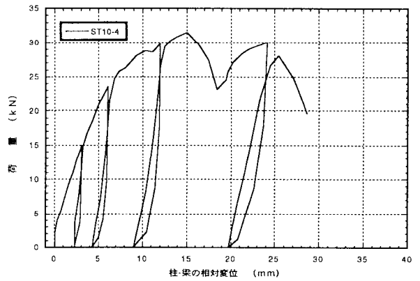
図4. 4 : ST10-4 7' 掛金物THF-10のせん断荷試験の荷重-変位曲線
