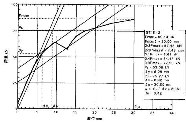
図 5. 2 : ST18-2 の荷重-変位包絡線
