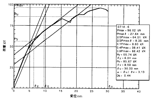
図 5. 6 : ST18-6 の荷重-変位包絡線
