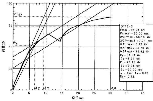
図 5. 3 : ST18-3 の荷重-変位包絡線
