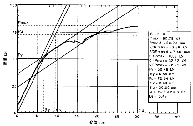
図 5. 4 : ST18-4 の荷重-変位包絡線
