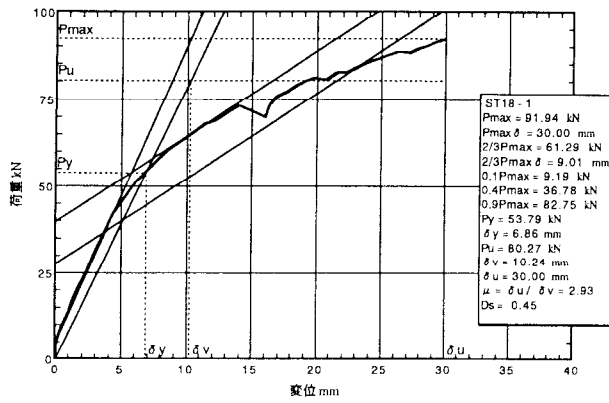
図 5. 1 : ST18-1 の荷重-変位包絡線
