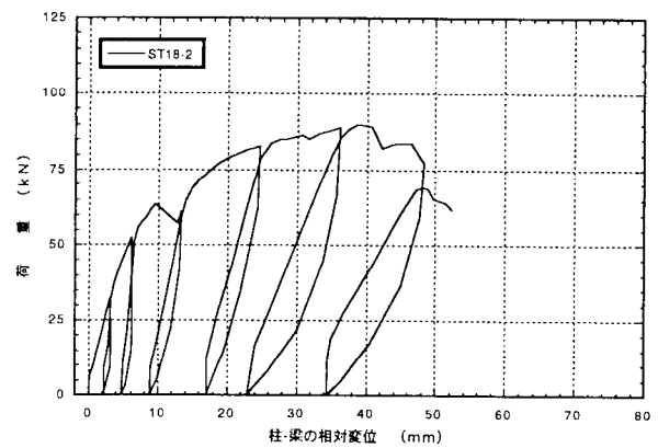
図4. 2 : ST18-2 7J 掛金物THF-18のせん断荷試験の荷重-変位曲線
