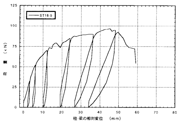
図4. 5 : ST18-5 7J 掛金物THF-18のせん断荷試験の荷重-変位曲線
