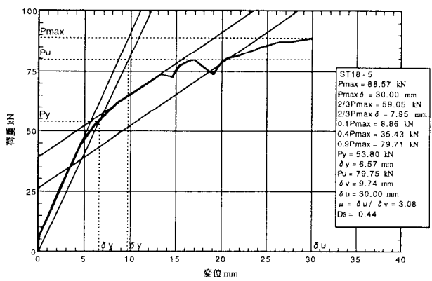
図 5. 5 : ST18-5 の荷重-変位包絡線
