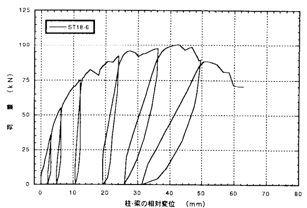
図4. 6 : ST18-6 7J 掛金物THF-18のせん断荷試験の荷重-変位曲線
