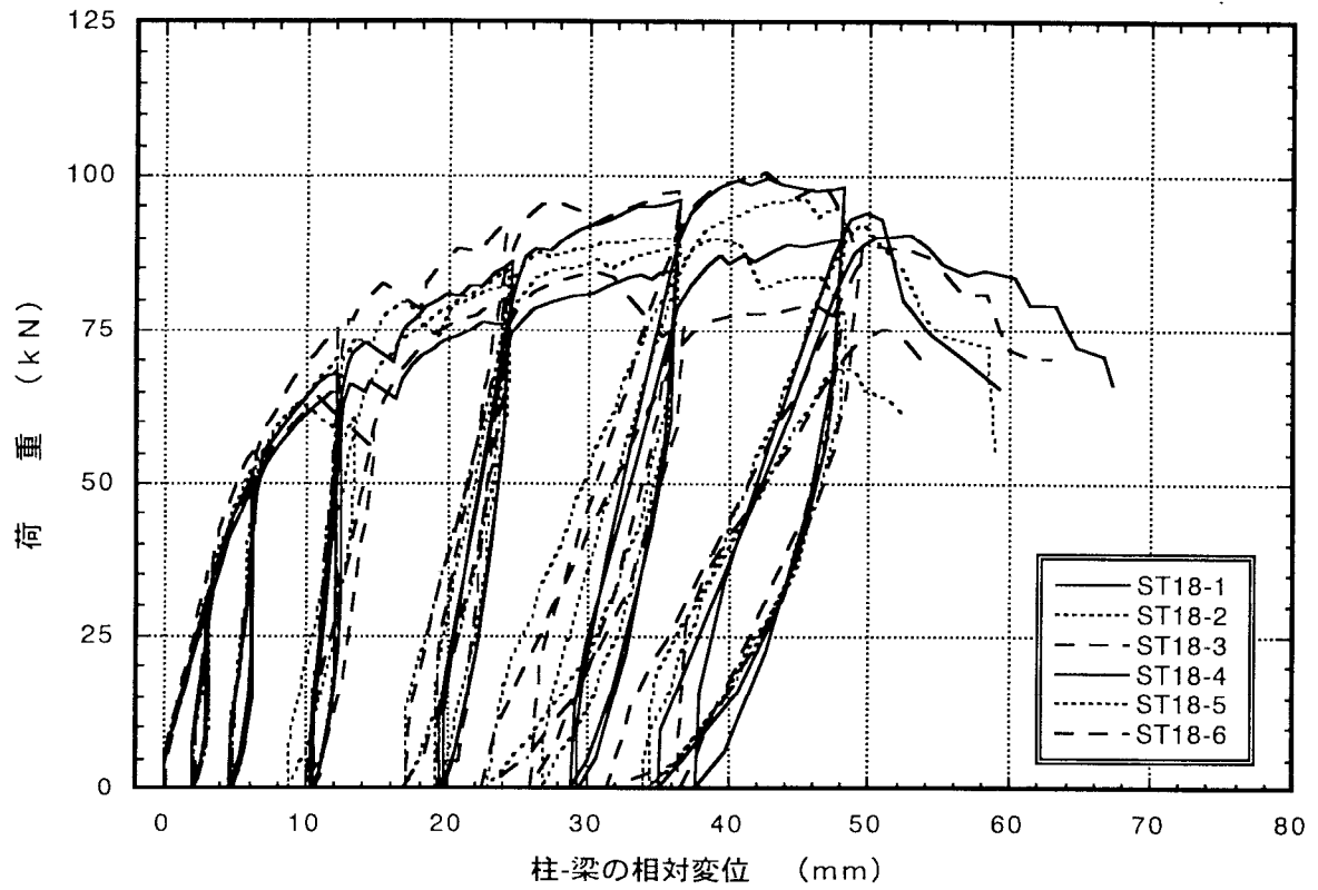
図4. 7 : ST18 7 角 掛金物THF-18のせん断載荷試験の荷重-変位曲線
