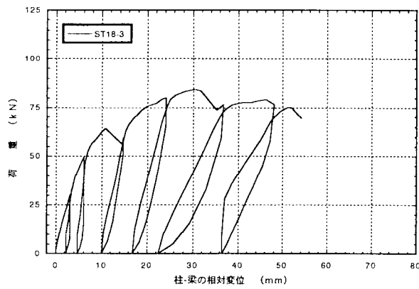
図4. 3 : ST18-3 7J 掛金物THF-18のせん断荷試験の荷重-変位曲線
