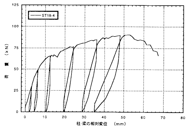
図4. 4 : ST18-4 7J 掛金物THF-18のせん断荷試験の荷重-変位曲線
