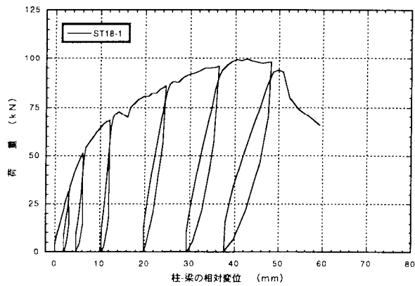
図4. 1 : ST18-1 7J 掛金物THF-18のせん断荷試験の荷重-変位曲線
