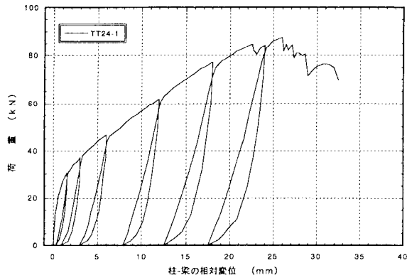
図4. 1 : TT24-1 アゴ掛金物THF-24の引張型載荷試験の荷重-変位曲線
