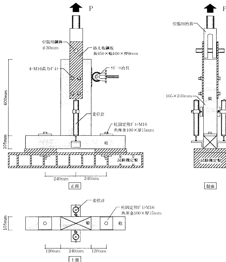
図3. 1：柱－梁接合部の引張型荷重試験方法
