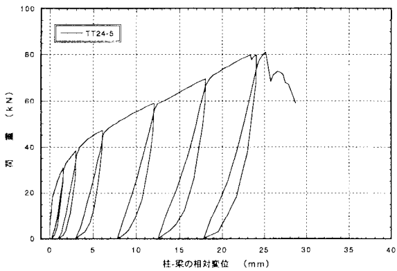
図4. 5 : TT24-5 アゴ掛金物THF-24の引張型載荷試験の荷重-変位曲線
