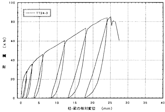
図4. 3 : TT24-3 アゴ掛金物THF-24の引張型載荷試験の荷重-変位曲線
