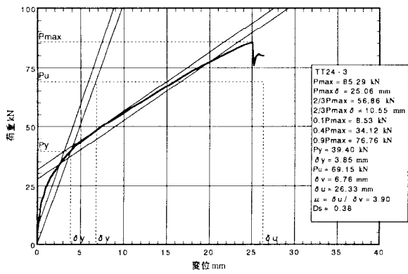
図5. 3 : TT24-3の荷重-変位包絡線
