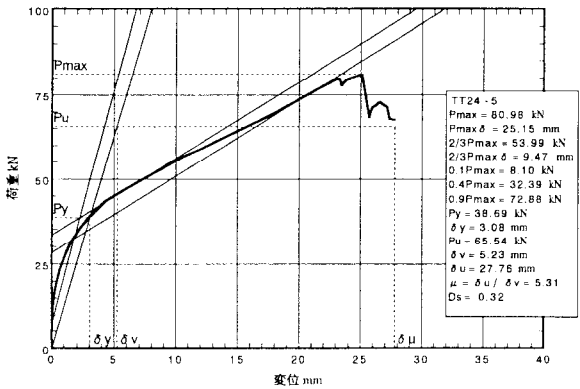
図5. 5 : TT24-5の荷重-変位包絡線
