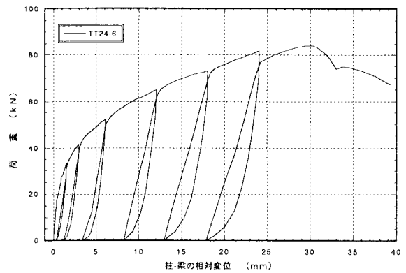
図4. 6 : TT24-6 アゴ掛金物THF-24の引張型載荷試験の荷重-変位曲線
