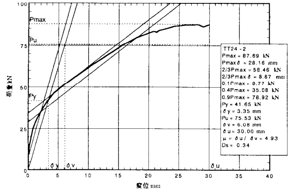
図5. 2 : TT24-2の荷重-変位包絡線
