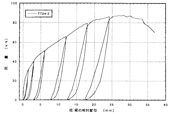
図4. 2 : TT24-2 アゴ掛金物THF-24の引張型載荷試験の荷重-変位曲線
