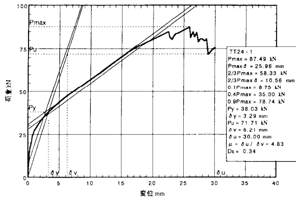
図5. 1 : TT24-1の荷重-変位包絡線
