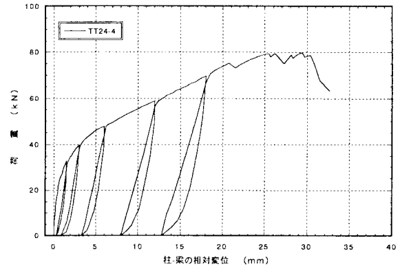
図4. 4 : TT24-4 アゴ掛金物THF-24の引張型載荷試験の荷重-変位曲線
