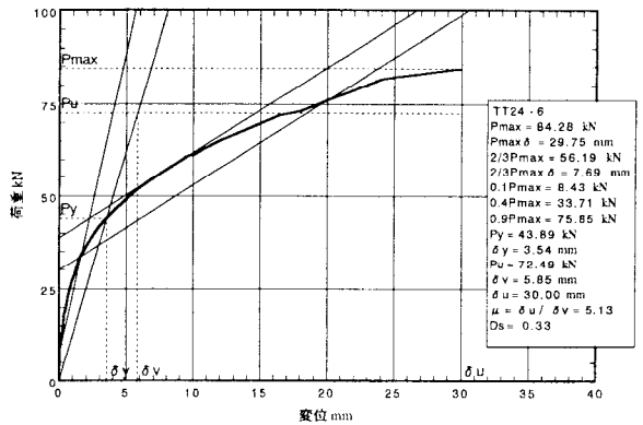
図5. 6 : TT24-6の荷重-変位包絡線
