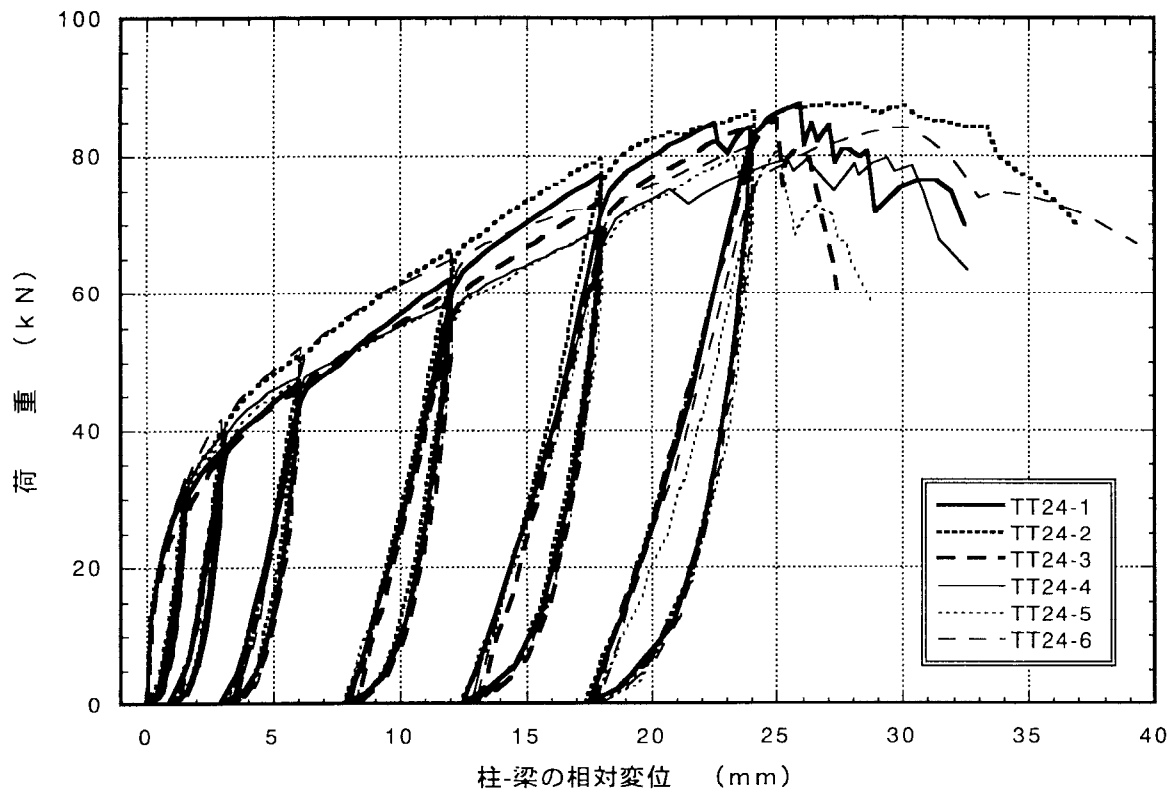
図4. 7 : TT24 アゴ掛金物THF-24の引張型載荷試験の荷重—変位曲線
