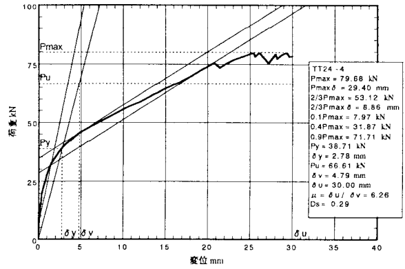
図5. 4 : TT24-4の荷重-変位包絡線
