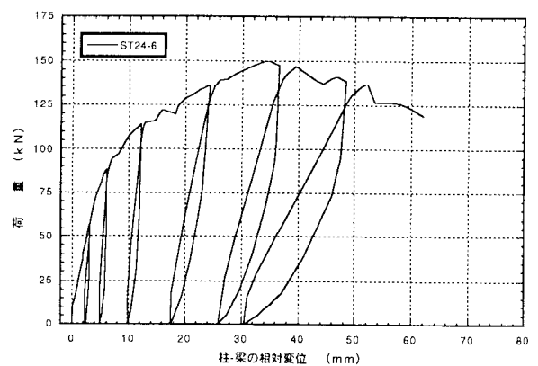
図4. 6 : ST24-6 70' 掛金物THF-24のせん断載荷試験の荷重-変位曲線
