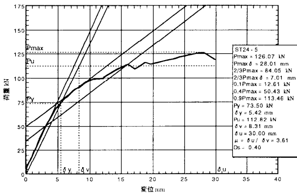
図5. 5 : ST 2 4-5の荷重-変位包絡線
