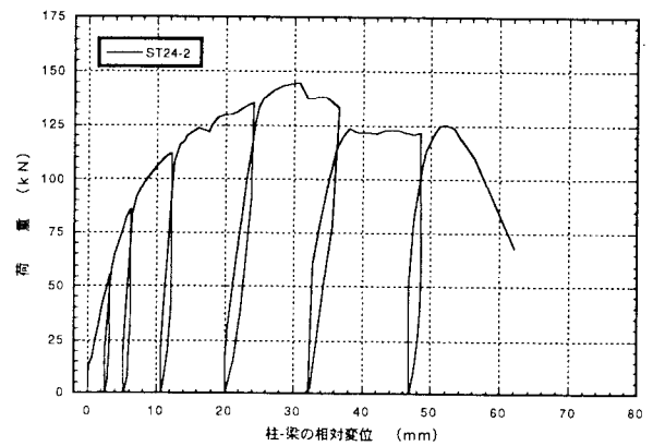
図4. 2 : ST24-2 70' 掛金物THF-24のせん断載荷試験の荷重-変位曲線
