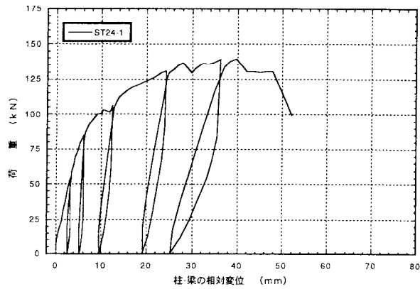
図4. 1 : ST24-1 70' 掛金物THF-24のせん断載荷試験の荷重-変位曲線
