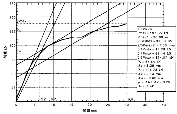
図5. 4 : ST 2 4-4の荷重-変位包絡線
