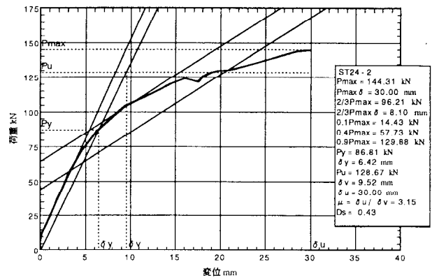
図5. 2 : ST 2 4-2の荷重-変位包絡線
