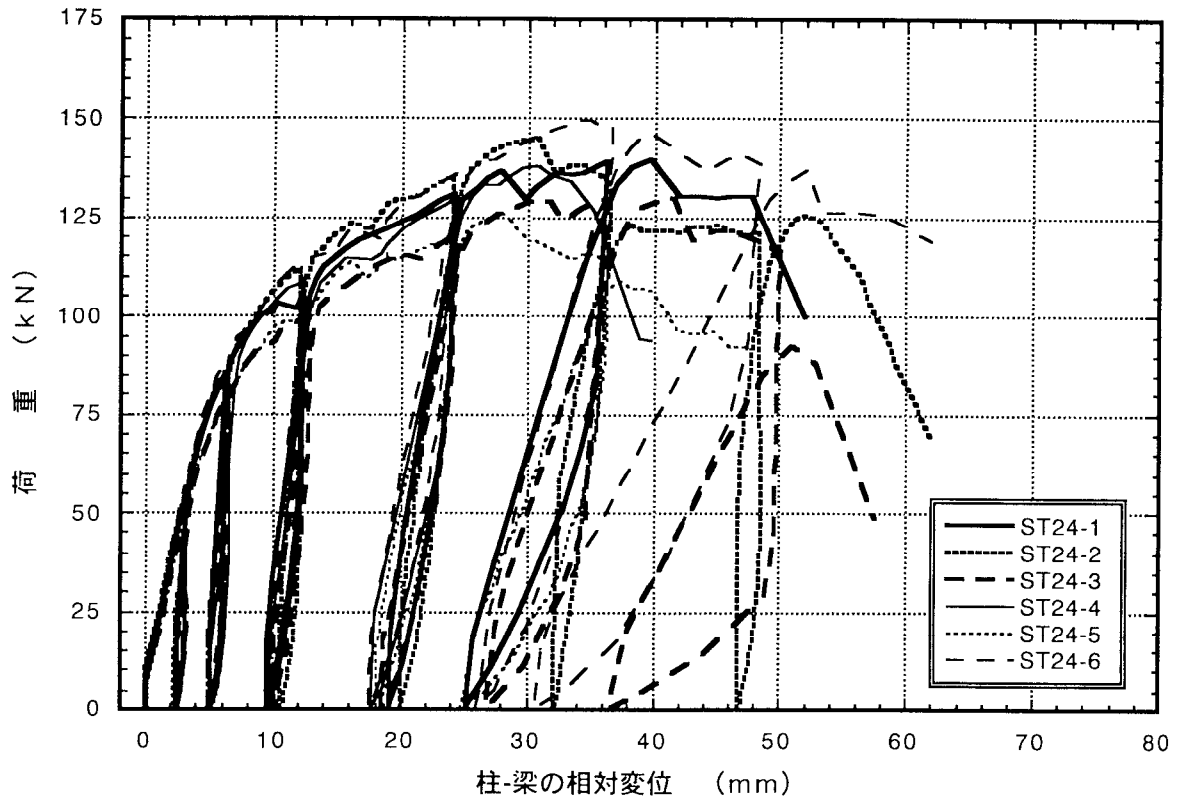
図4. 7 : ST24 7J' 掛金物THF-24のせん断載荷試験の荷重-変位曲線
