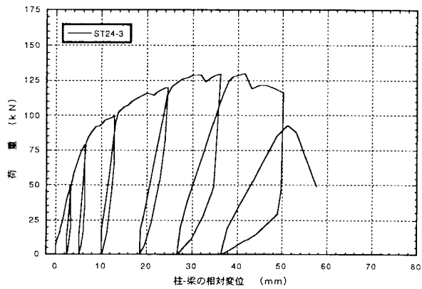
図4. 3 : ST24-3 70' 掛金物THF-24のせん断載荷試験の荷重-変位曲線
