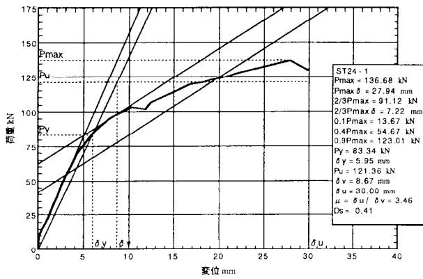
図5. 1 : ST 2 4-1の荷重-変位包絡線
