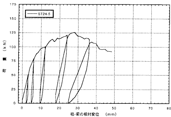
図4. 5 : ST24-5 70' 掛金物THF-24のせん断載荷試験の荷重-変位曲線
