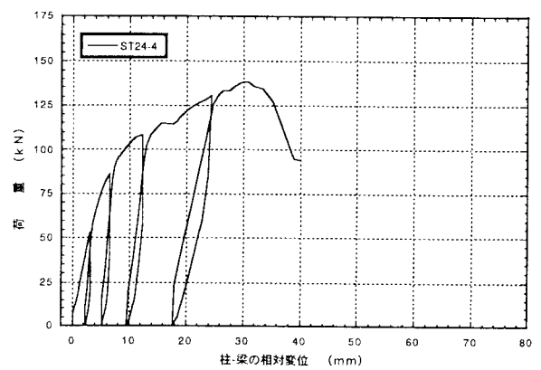
図4. 4 : ST24-4 70' 掛金物THF-24のせん断載荷試験の荷重-変位曲線
