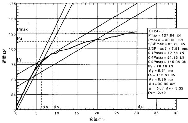
図5. 3 : ST 2 4-3の荷重-変位包絡線
