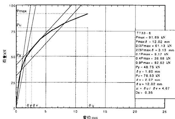
図5. 6 : TT33-6の荷重-変位包絡線
