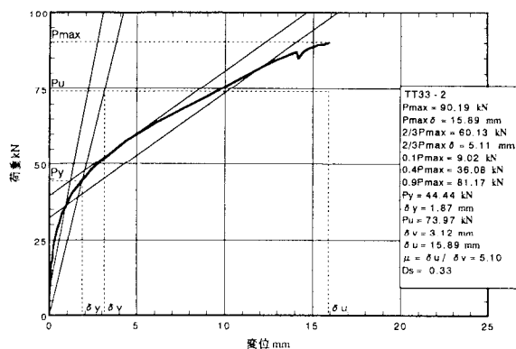
図5. 2 : TT33-2の荷重-変位包絡線
