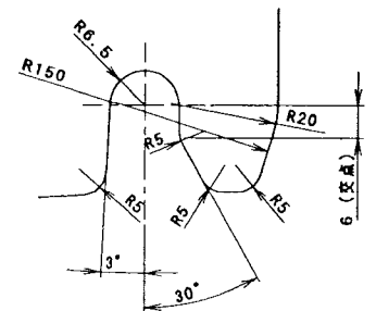
D部詳細図 (S=2/3)
