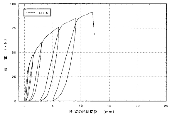
図4. 6 : TT33-6 アゴ掛金物THF-33の引張型載荷試験の荷重-変位曲線
