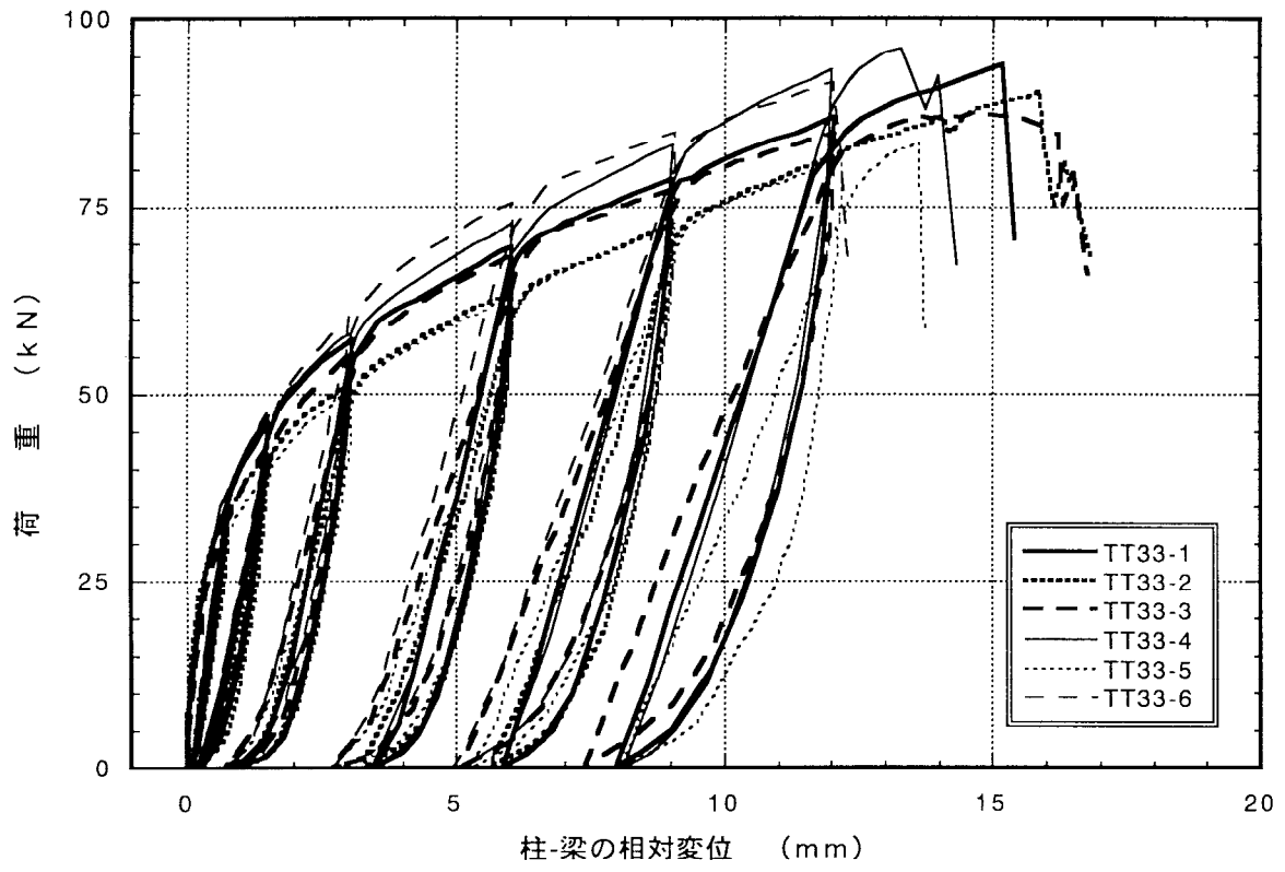
図4. 7 : TT33 アゴ掛金物THF-33の引張型載荷試験の荷重-変位曲線
