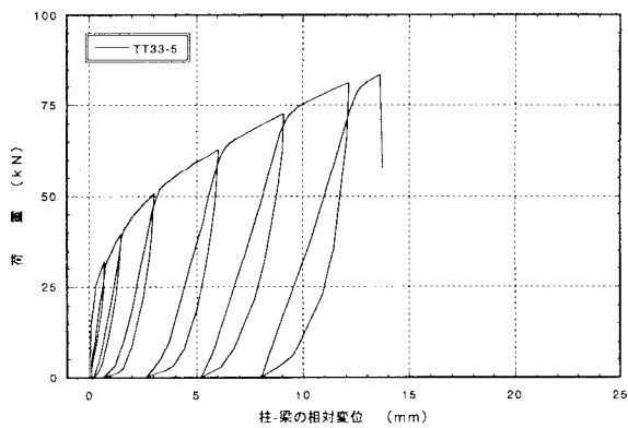
図4. 5 : TT33-5 アゴ掛金物THF-33の引張型載荷試験の荷重-変位曲線
