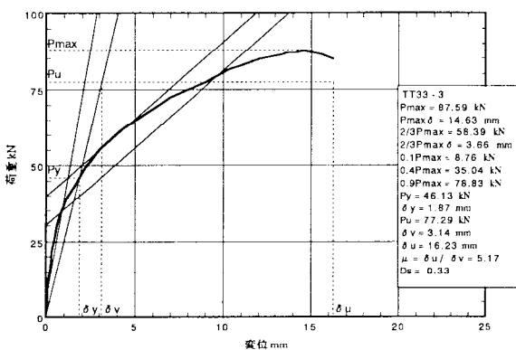
図5. 3 : TT33-3の荷重-変位包絡線
