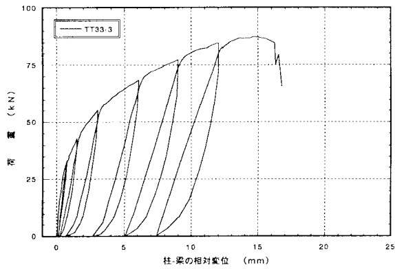
図4. 3 : TT33-3 アゴ掛金物THF-33の引張型載荷試験の荷重-変位曲線
