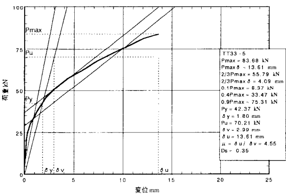
図5. 5 : TT33-5の荷重-変位包絡線
