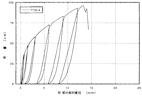
図4. 4 : TT33-4 アゴ掛金物THF-33の引張型載荷試験の荷重-変位曲線
