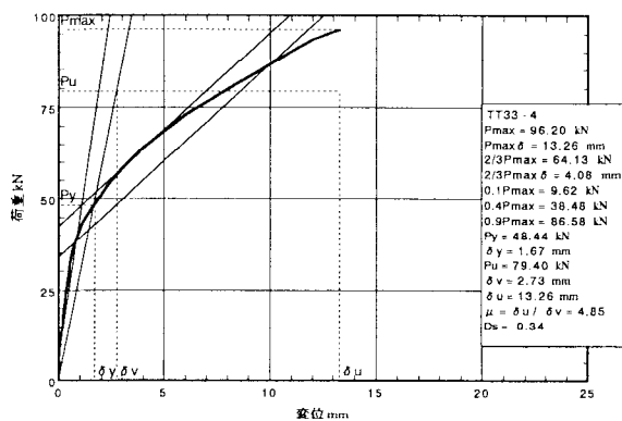
図5. 4 : TT33-4の荷重-変位包絡線
