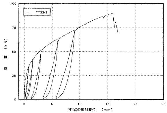
図4. 2 : TT33-2 アゴ掛金物THF-33の引張型載荷試験の荷重-変位曲線
