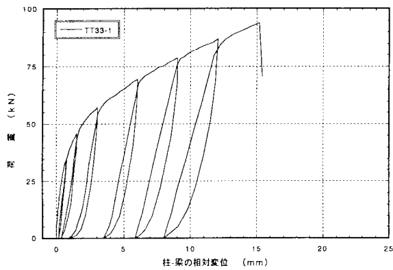
図4. 1 : TT33-1 アゴ掛金物THF-33の引張型載荷試験の荷重-変位曲線
