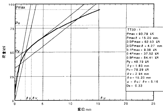
図5. 1 : TT33-1の荷重-変位包絡線
