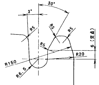
C部詳細図 (S=2/3)
