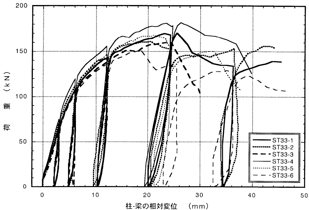
図4. 7 : ST33 7J 1 掛金物THF-33のせん断載荷試験の荷重-変位曲線
