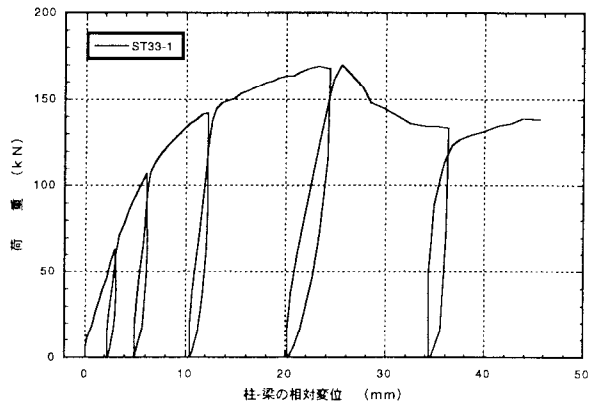
図4. 1 : ST33-1 70' 掛金物THF-33のせん断載荷試験の荷重-変位曲線
