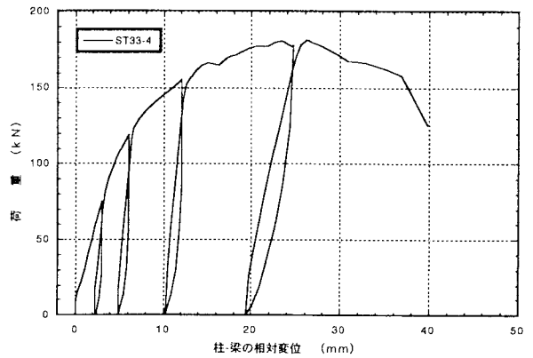
図4. 4 : ST33-4 70' 掛金物THF-33のせん断載荷試験の荷重-変位曲線
