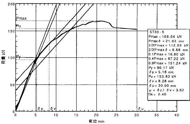
図 5. 5 : ST 3 3-5 の荷重-変位包絡線
