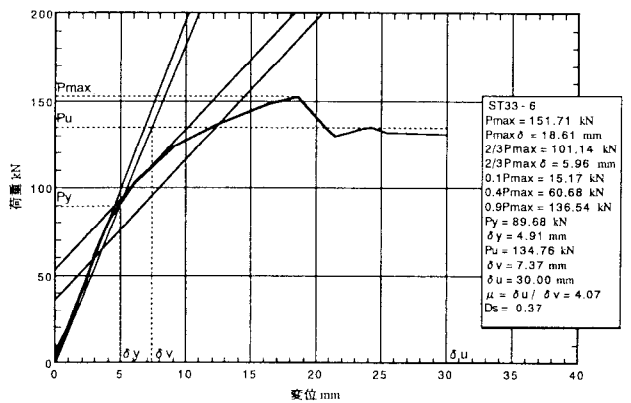
図 5. 6 : ST 3 3-6 の荷重-変位包絡線
