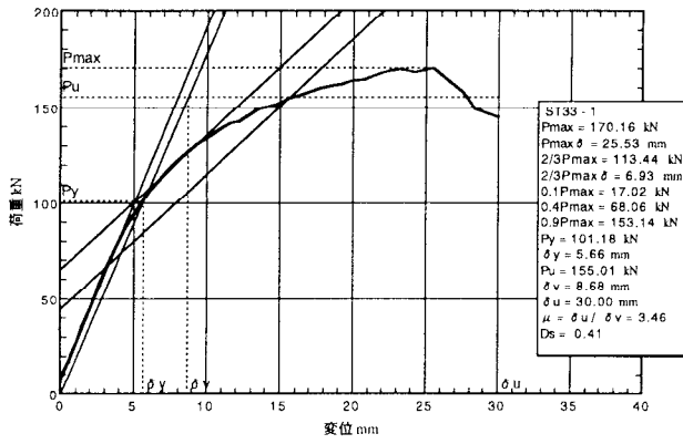
図 5. 1 : ST 3 3-1 の荷重-変位包絡線
