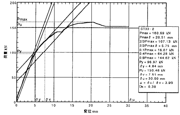
図 5. 2 : ST 3 3-2 の荷重-変位包絡線
