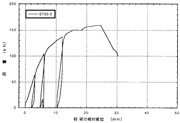
図4. 3 : ST33-3 70' 掛金物THF-33のせん断載荷試験の荷重-変位曲線
