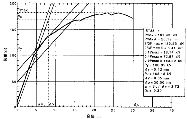
図 5. 4 : ST 3 3-4 の荷重-変位包絡線
