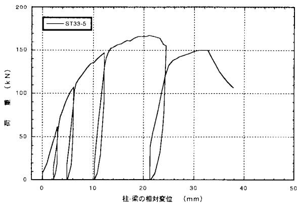
図4. 5 : ST33-5 70' 掛金物THF-33のせん断載荷試験の荷重-変位曲線
