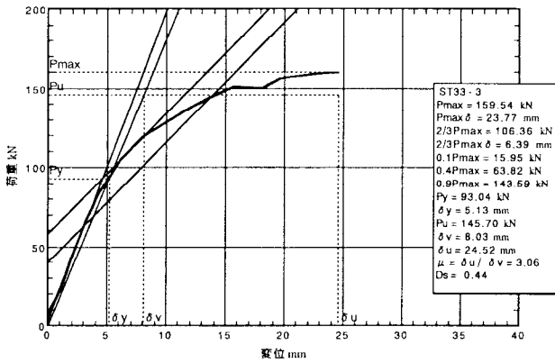
図 5. 3 : ST 3 3-3 の荷重-変位包絡線
