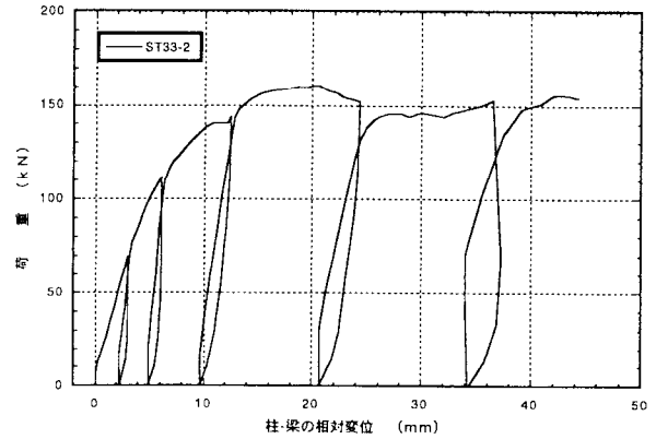
図4. 2 : ST33-2 70' 掛金物THF-33のせん断載荷試験の荷重-変位曲線
