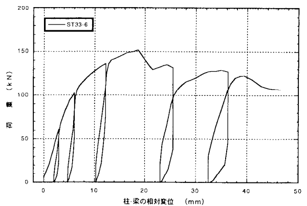
図4. 6 : ST33-6 70' 掛金物THF-33のせん断載荷試験の荷重-変位曲線
