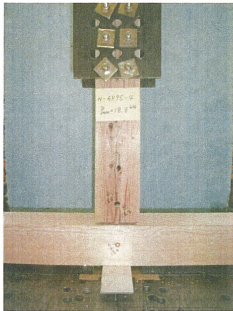
写真-4 破壊状況
