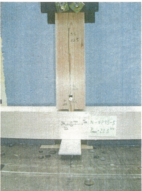
写真-5 破壊状況
