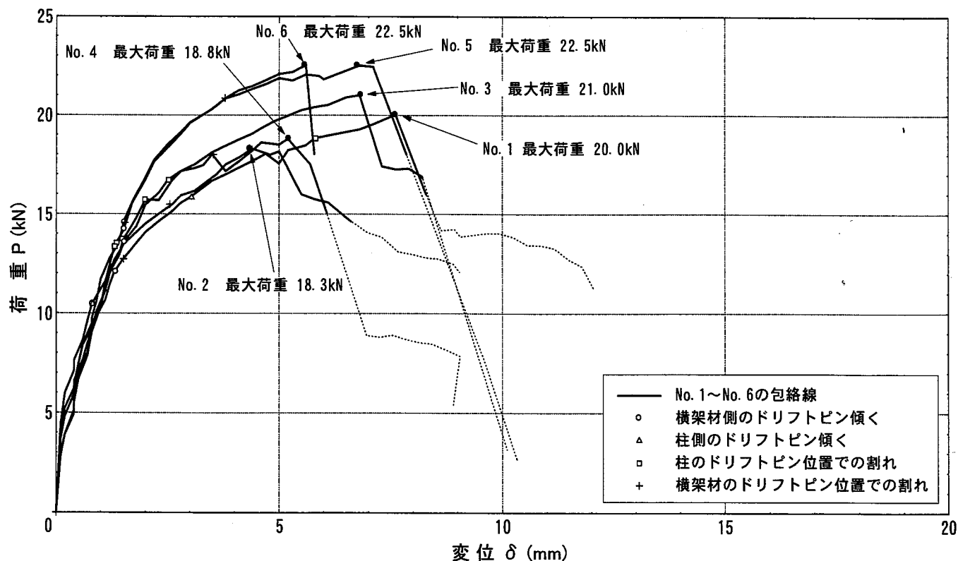
図-3 荷重 - 変位 包絡線の比較
