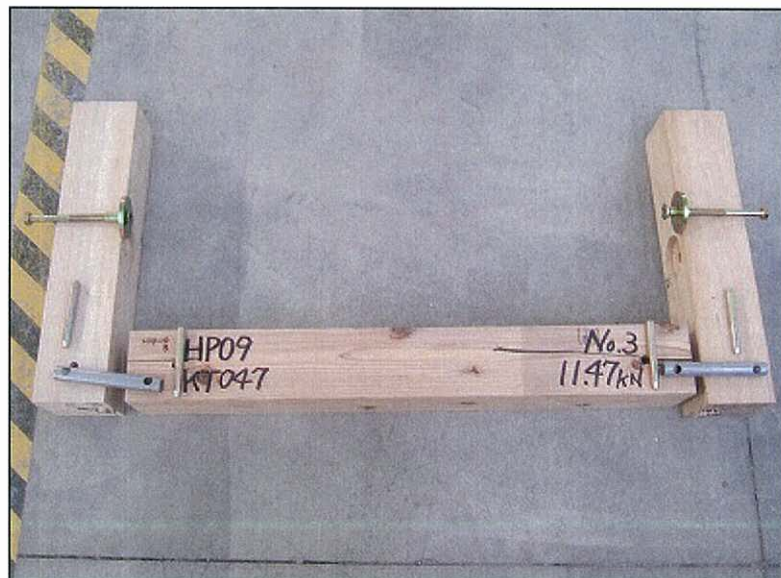
写真 3(3) 終局状況 (No.3)
