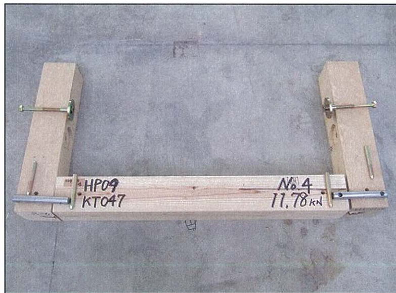
写真 4(3) 終局状況 (No.4)
