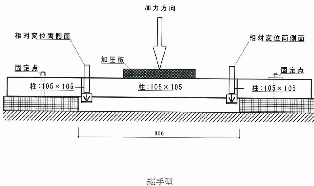
図 3.1 継手型試験体とせん断試験方法(概念図)
