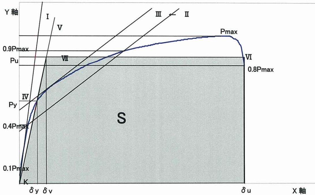
図 4.1 完全弾塑性モデルによる降伏耐力、終局耐力等の求め方
