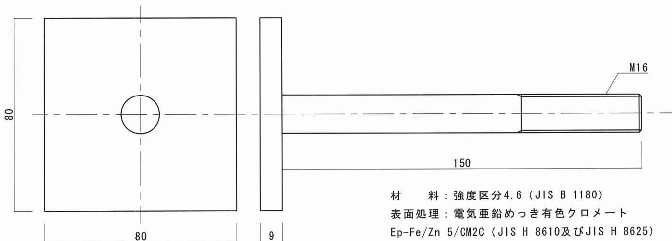
図2.3 接合具
