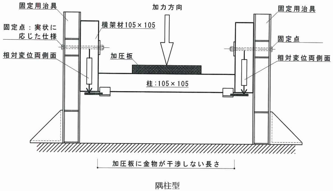
図 3.1 隅柱型試験体とせん断試験方法(概念図)
