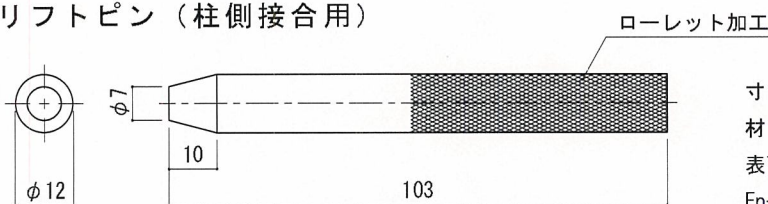
接合具 図2.3
