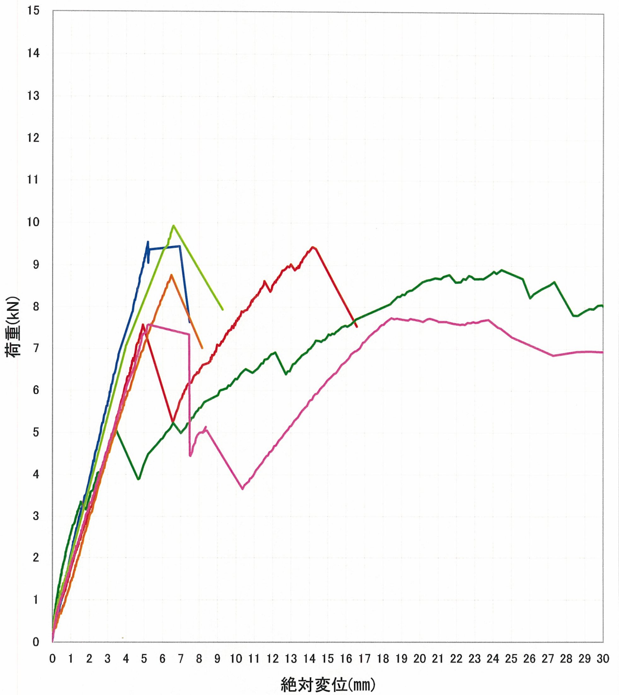
荷重-変位関係包絡線一覧
