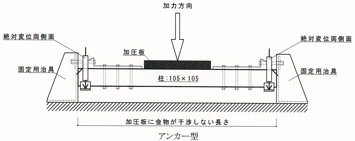
図 3.1 アンカー型試験体とせん断試験方法(概念図)
