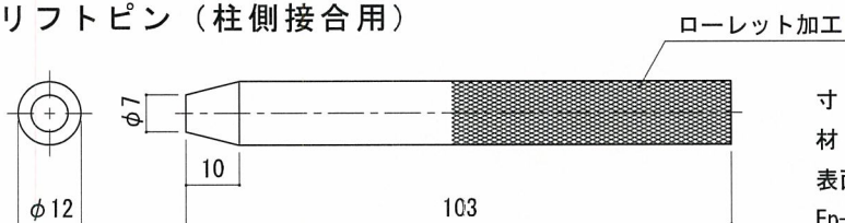
接合具 図2.3
